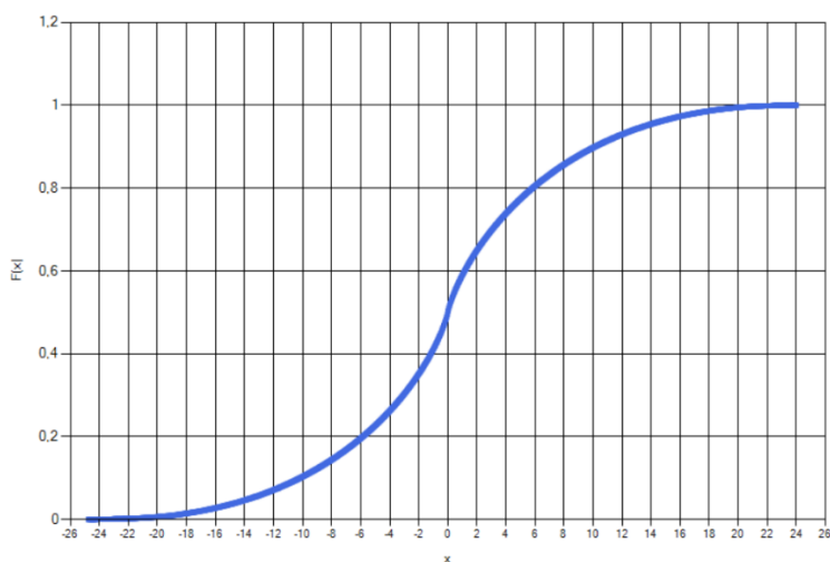
Рис. 2. График функции распределения произведения двух стандартных нормальных случайных величин
