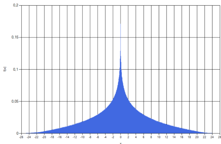
Рис. 1. График функции плотности произведения двух стандартных нормальных распределений
