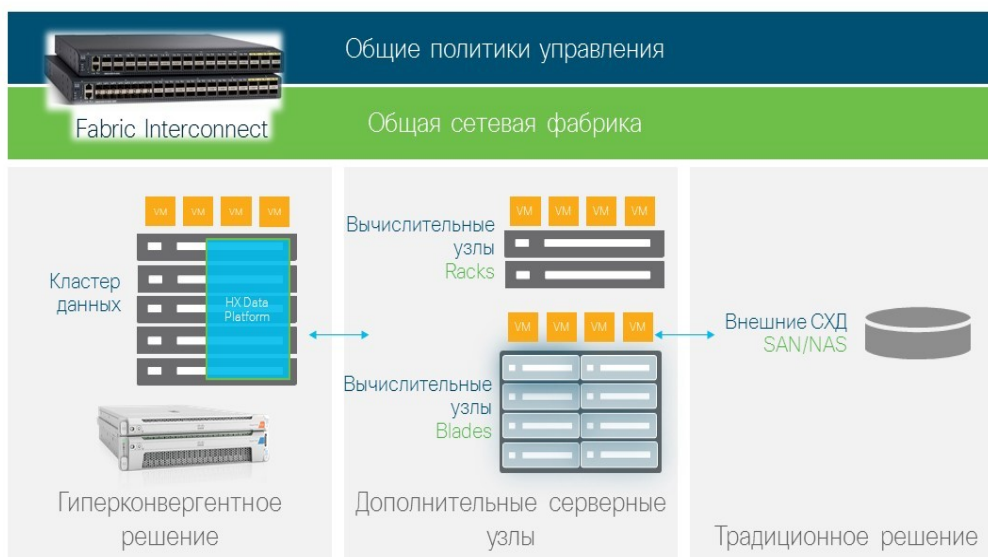
Рис. Общая схема кластера Hyperflex с обозначением всех указанных компонентов
