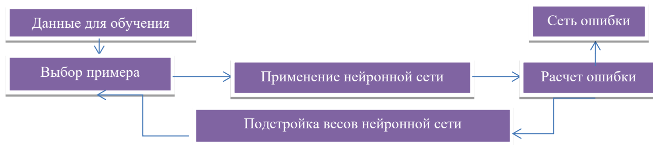
Рис. 2. Упрощенный алгоритм процесса обучения нейронной сети
