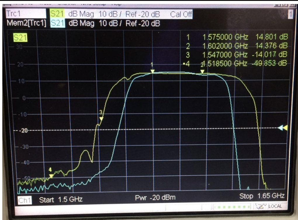
Рис. 7. Сравнение передаточных характеристик антенн
