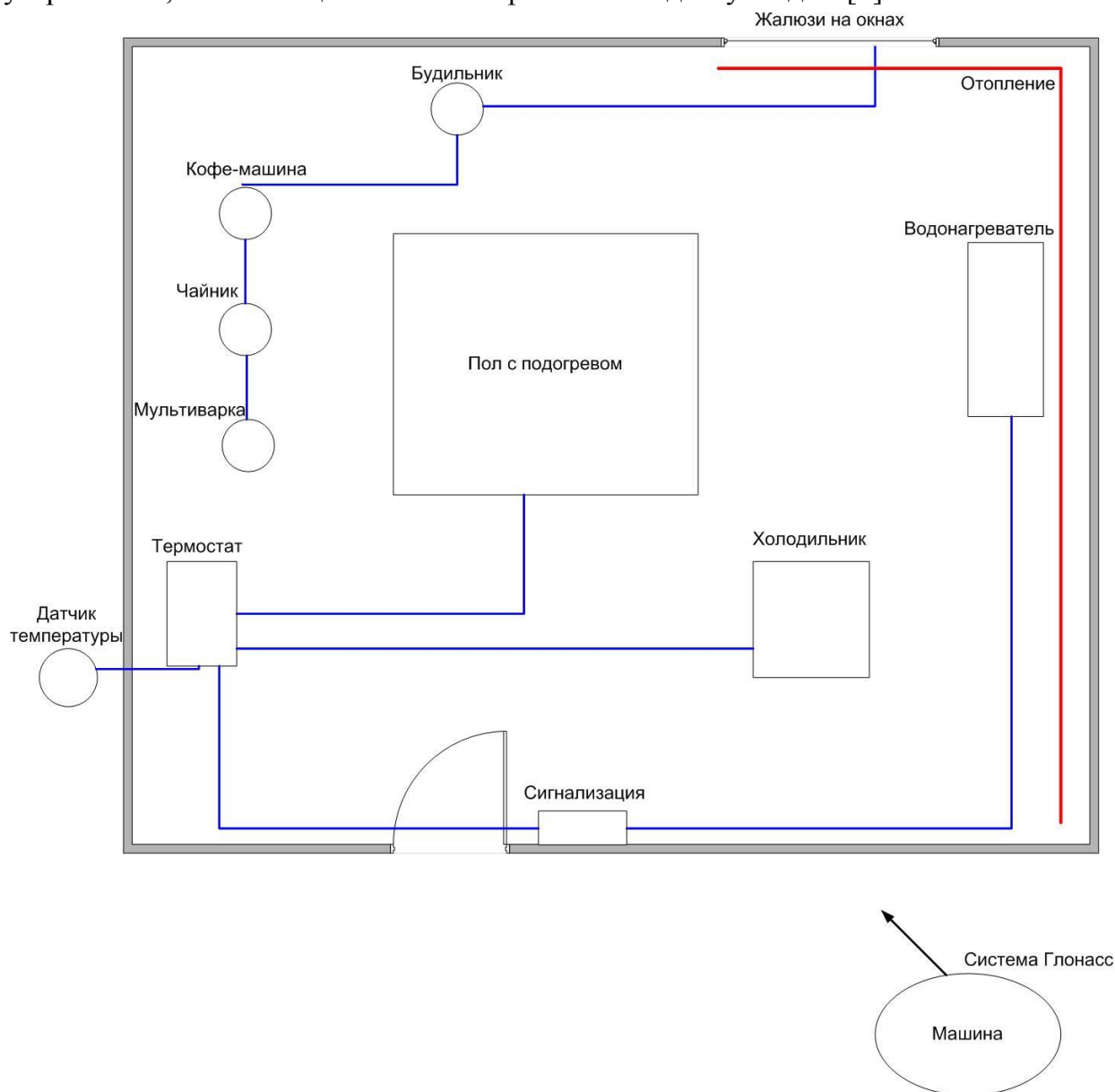
Рис. Структурная схема «умного» дома
