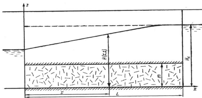
Рис. 2. Схема к расчету напоров в трещиноватом пласте при работе в нем прямолинейной совершенной граншеи
