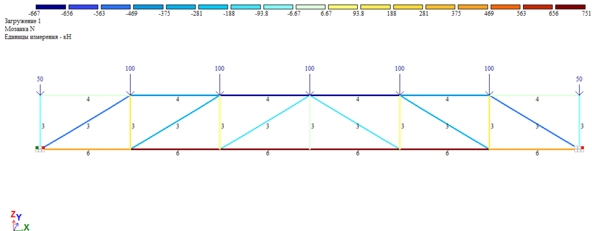
Рис. 1. Мозаика продольных сил N
