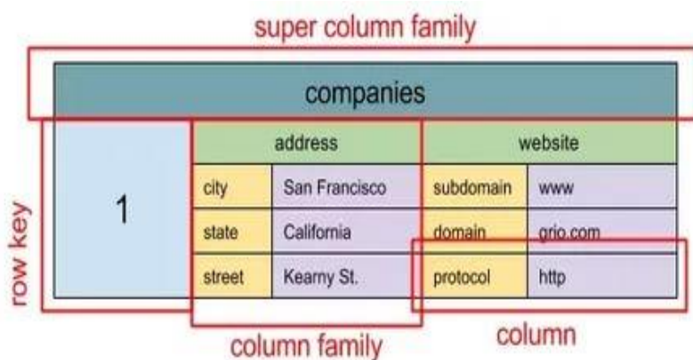
Рис. 6. Упрощенное представление данных Wide-column store
