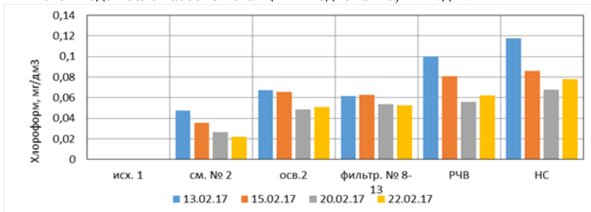
Рис. 1. Динамика изменения содержания хлороформа по стадиям очистки: исх.1 – природная вода; см. № 2 – после смесителя; осв.2 – после отстойника; фильтр. № 8-13 – после фильтрования; РЧВ – после резервуара чистой воды; НС – подача воды в распределительную сеть
