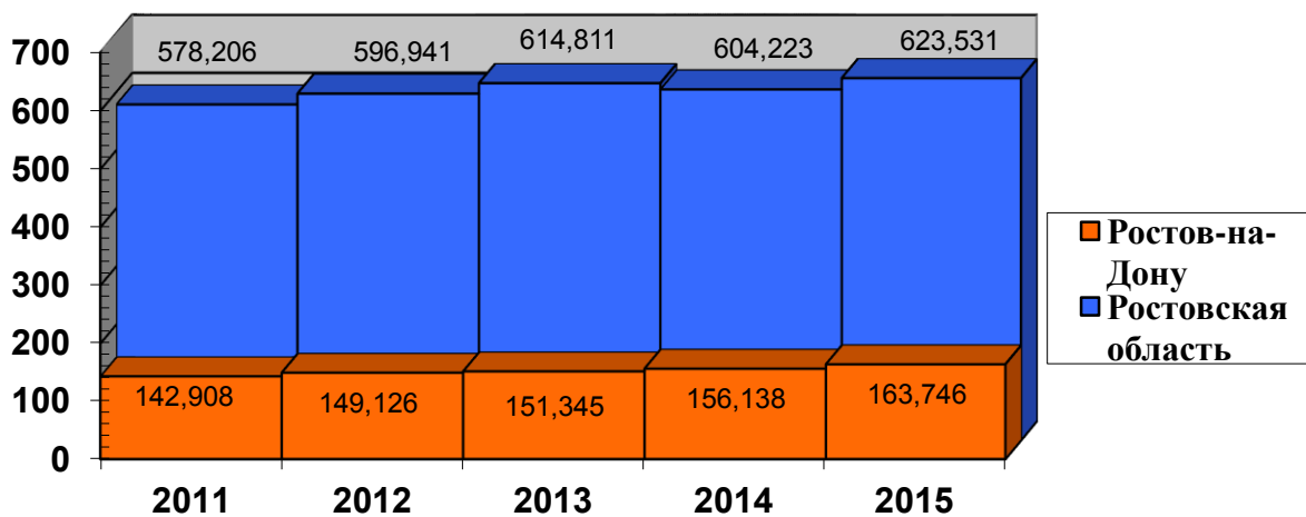
Рис. 2. Динамика валовых выбросов загрязняющих веществ в атмосферу от автотранспорта в Ростовской области (тыс. тонн) за 2010-2015 годы и их доля приходящаяся на город Ростов-на-Дону
