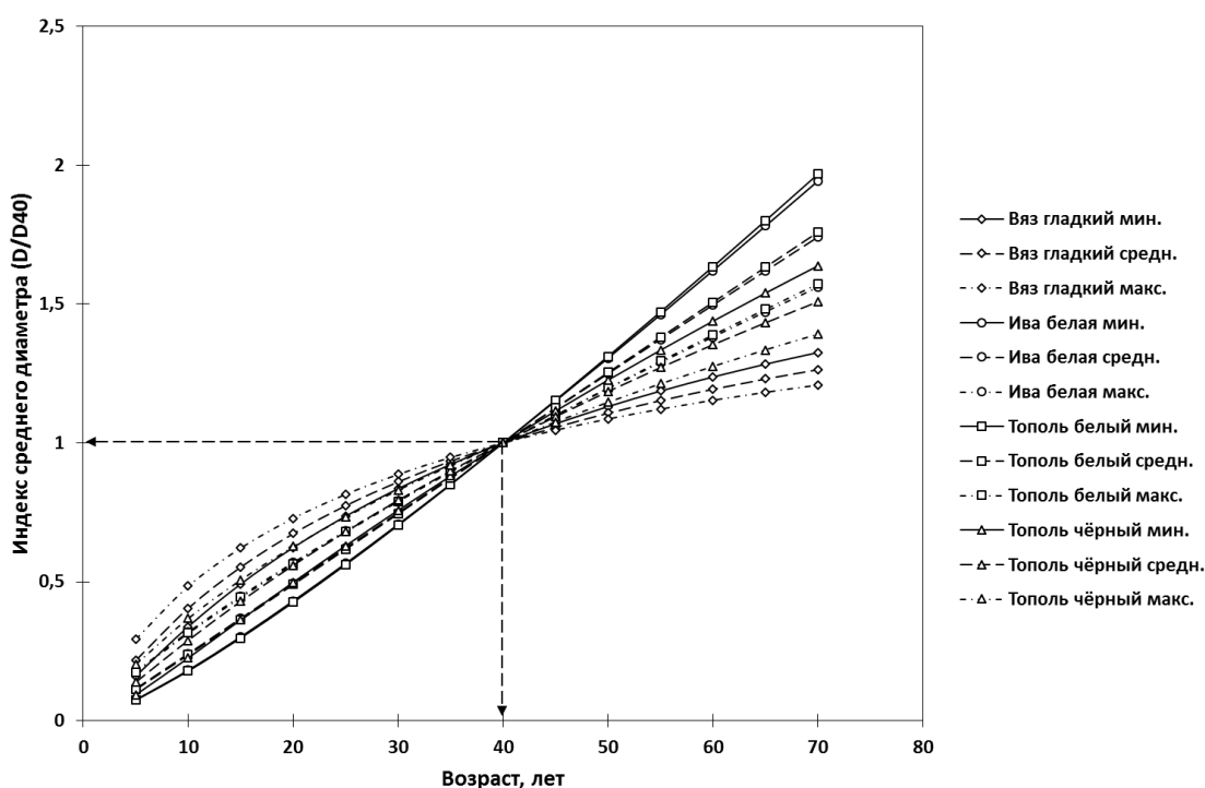
Рис. 4. Индексные кривые хода роста средних диаметров в смешанных древостоях ТБСЦ
