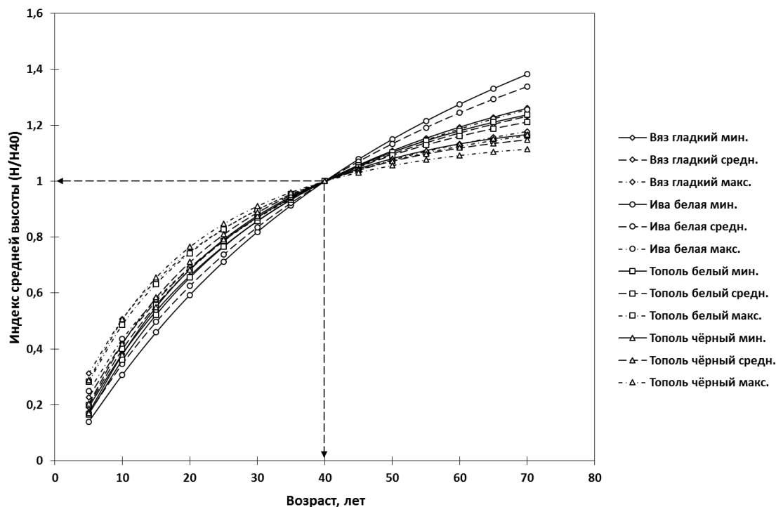
Рис. 2. Индексные кривые хода роста средних высот в смешанных древостоях ТБСЦ
