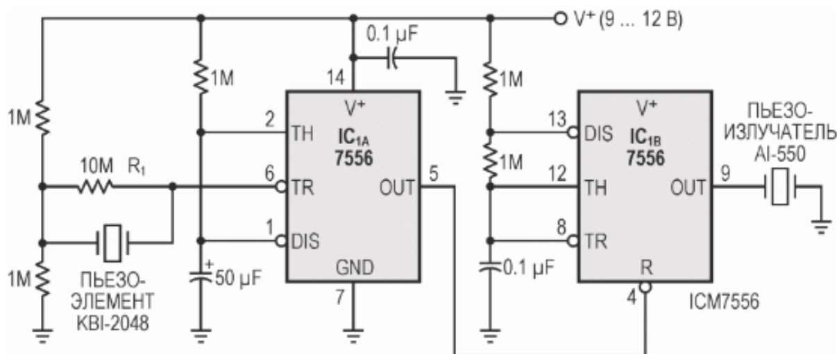
Рис. 3. Схема работы датчика удара
