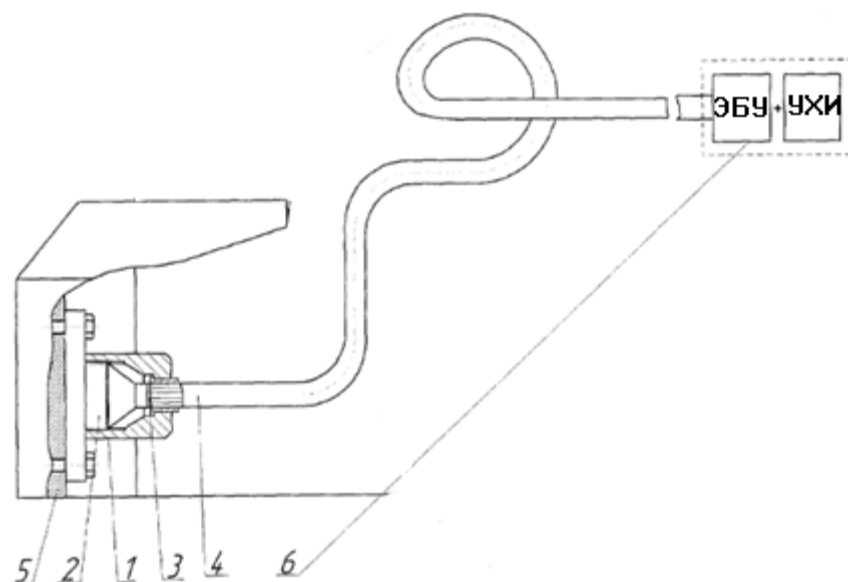
Рис. 4. Устройство механолуминесцентного датчика удара
