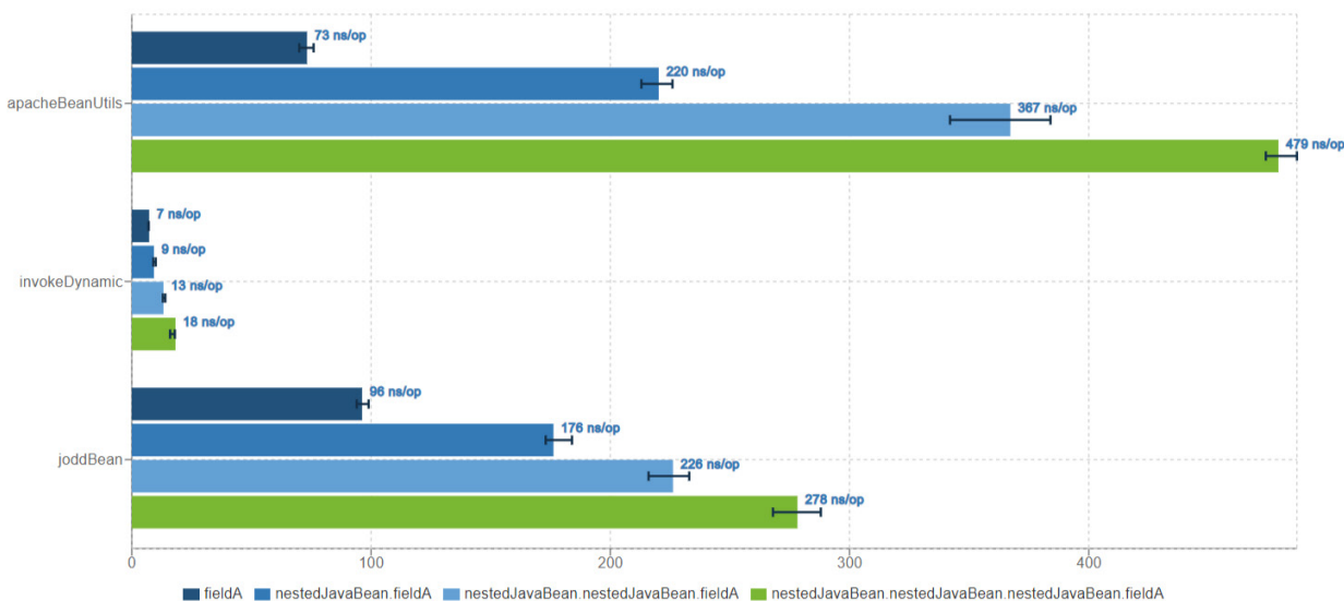
Рис. 3. Результаты GraalVM EE 1.0.0-rc9
