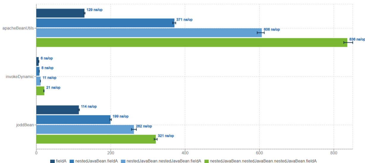
Рис. 2. Результаты Oracle JDK 8u191
