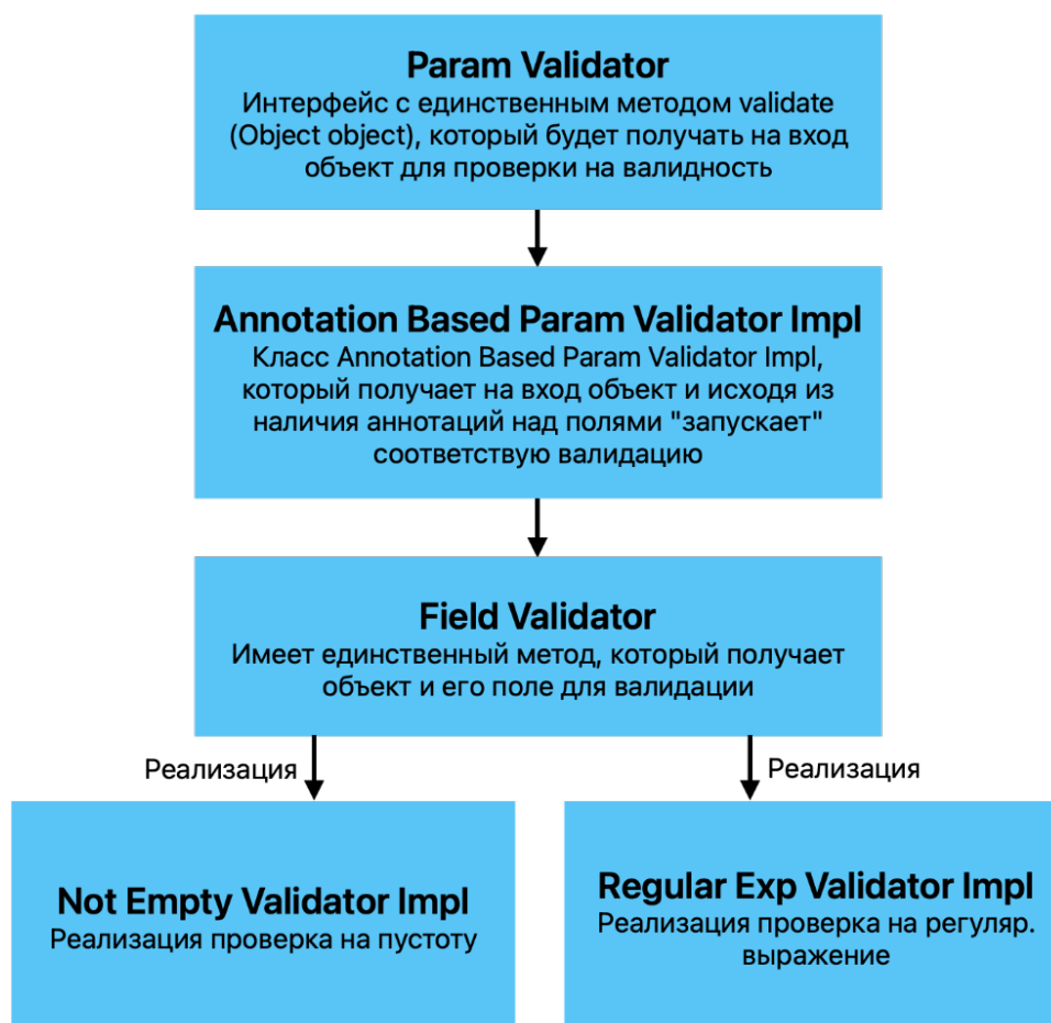
Рис. 1. Интерфейс ParamValidator
