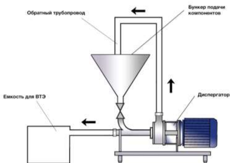
Рис. 2. Схема работы оборудования
