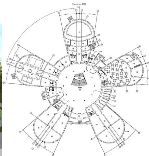
Рис. 1. Проект начальная школы на 200 мест в Нижнем Новгороде: а – визуализация; б – план на отм. 0.000
