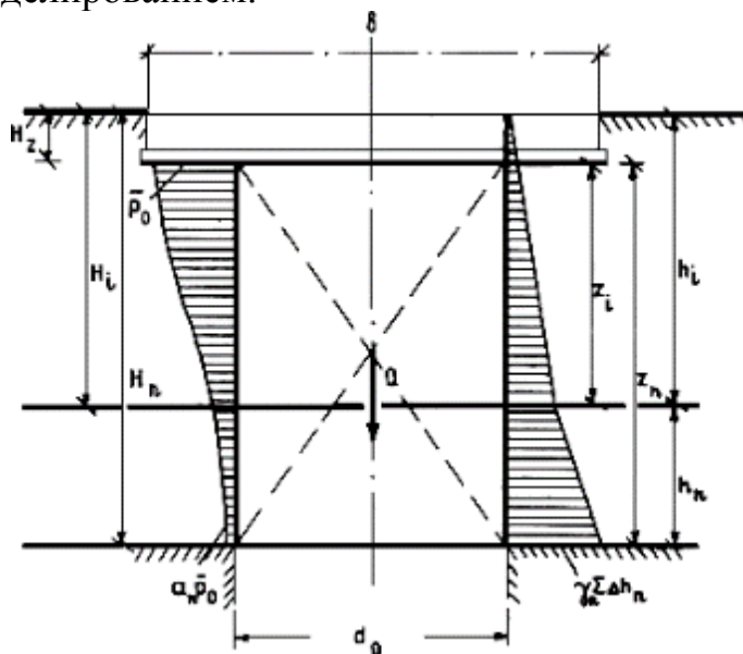
Рис. 1. Классическая расчетная схема для определения диаметра карстового провала
