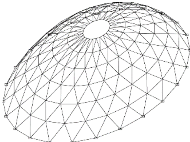
Рис. 1. Конечно-элементная модель купола кругового очертания
