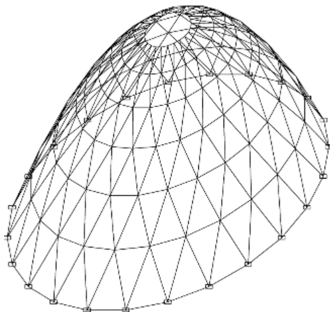
Рис. 2. Конечно-элементная модель купола параболического очертания
