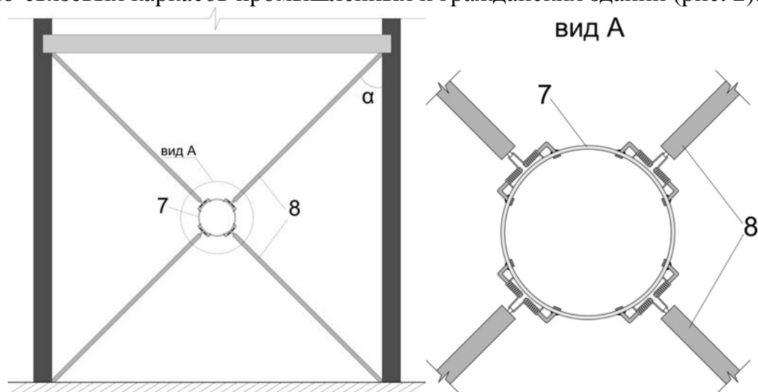
Рис. 2. КДГКТТ в крестовых связях: 7 – кольцо, 8 – связи
