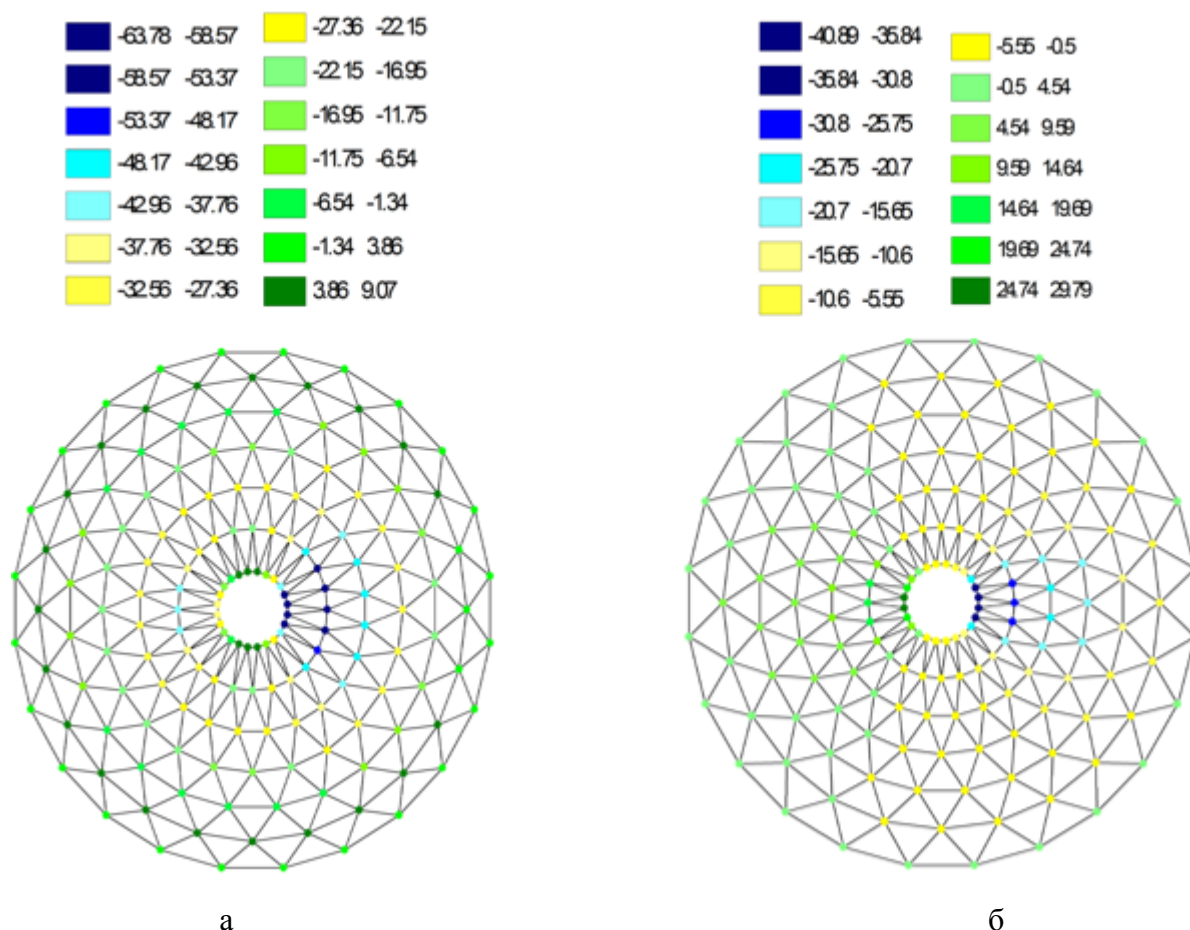
Рис. 3. Вертикальные перемещения (прогибы), мм; а – в куполе кругового очертания, б – в куполе параболического очертания
