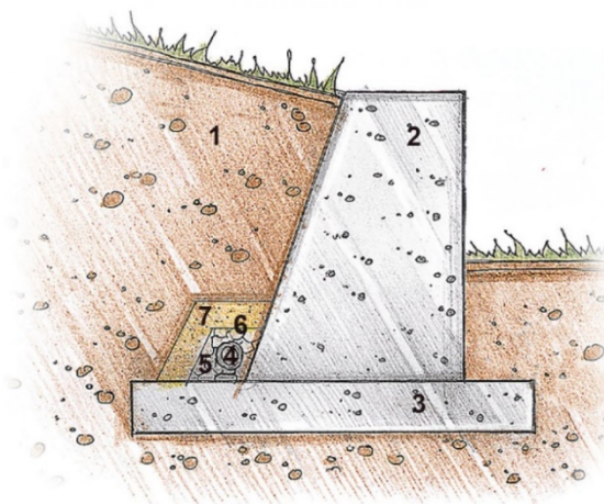
Рис. 1. Массивная подпорная стенка
