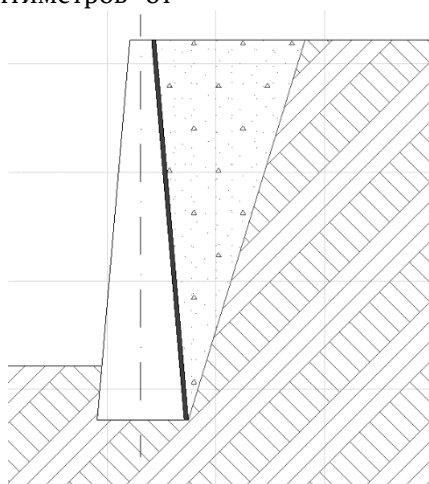
Рис. 2. Трапециевидная подпорная стенка
