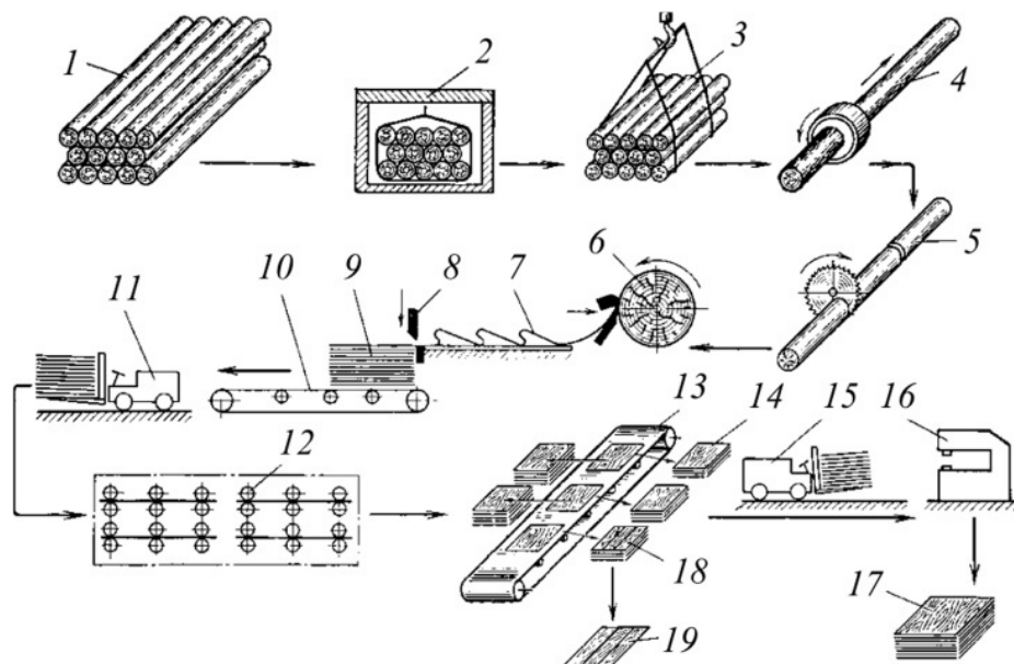
Рис. Схема технологического производства лущеного шпона [2]: 1 – склад сырья; 2 – гидротермическая обработка сырья; 3 – транспортировка сырья на участок подготовки; 4, 5 – подготовка сырья; 6 – лущение; 7 – лента лущеного шпона; 8 – раскрой шпона на ножницах; 9 – формирование пакета; 10 – конвейер выкатки патов из-под ножниц; 11, 15 – автопогрузчики; 12 – сушка шпона; 13 – сортировка шпона; 14 – формирование пакета из полноформатных листов шпона; 16 – починка шпона; 17 – формирование пакета из полноформатных листов шпона после починки; 18 – кусковые листы шпона; 19 – склеивание кускового шпона
