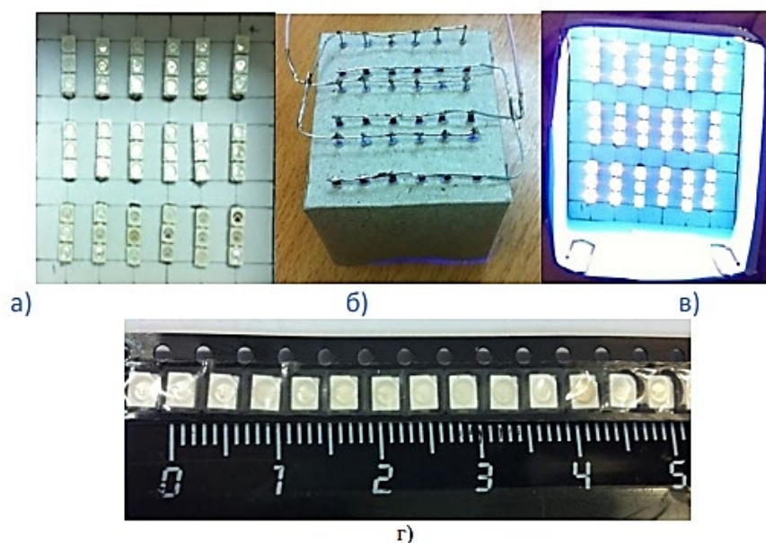
Рис. 1. Расположение УФ светодиодов в облучательной установке а) расположение УФ LED; б) крепление и пайка УФ LED; в) включенные УФ LED; г) размеры используемых УФ LED
