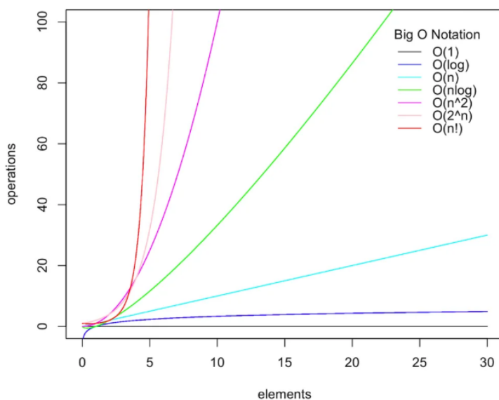
Рис. 6. График зависимости числа элементов от числа операций
