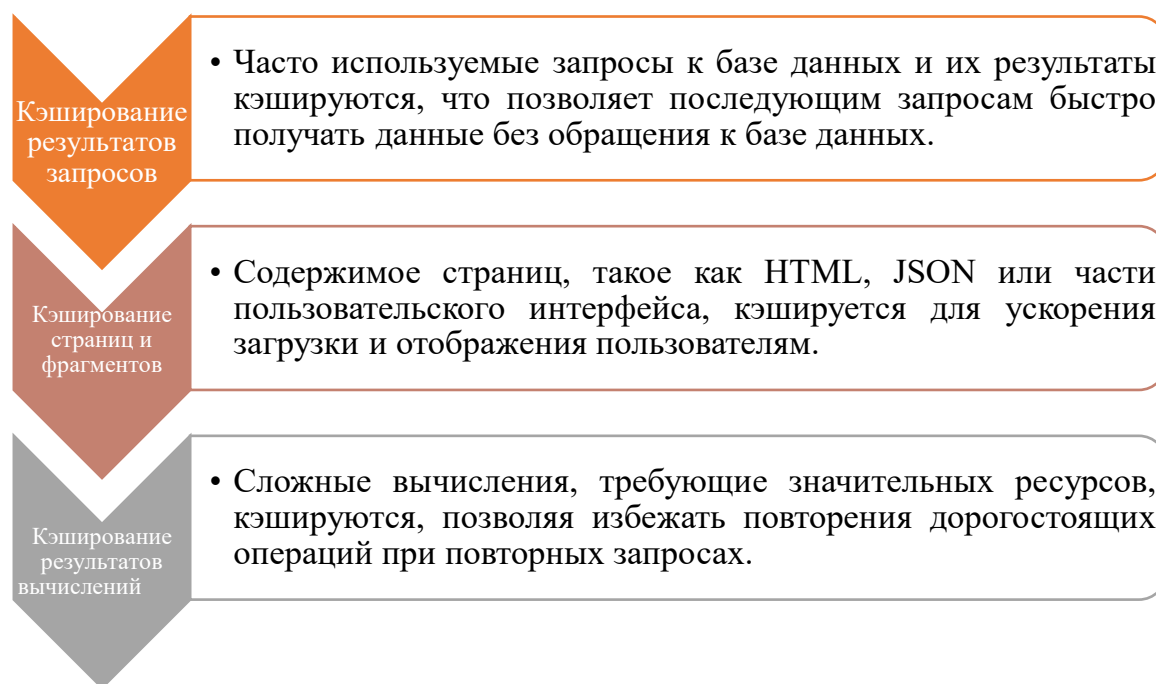
Рис. 1. Применение кэширования в веб-приложениях с Redis
