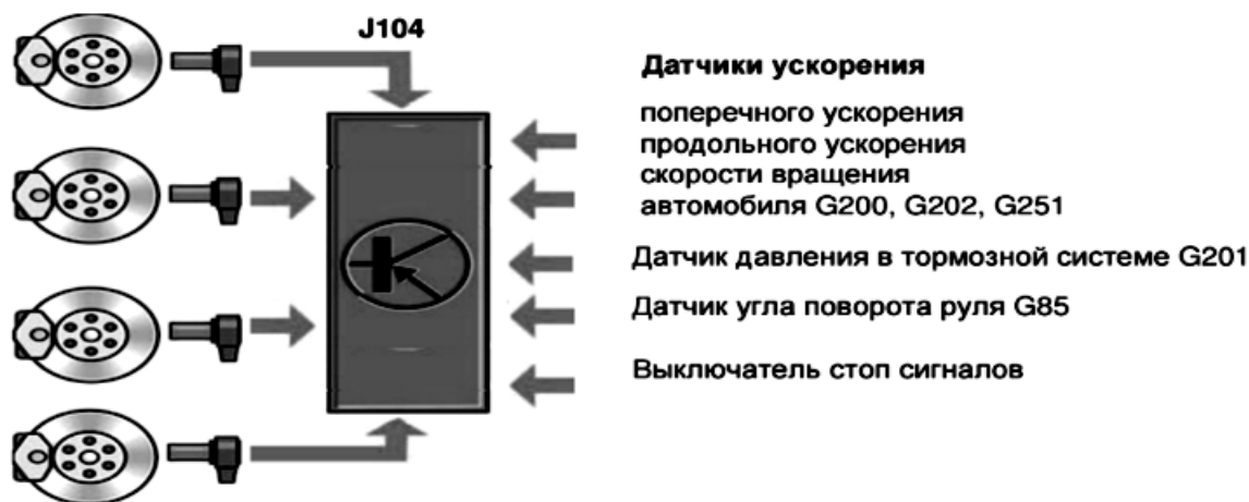
Рис. 2. Принцип работы датчиков ускорения
