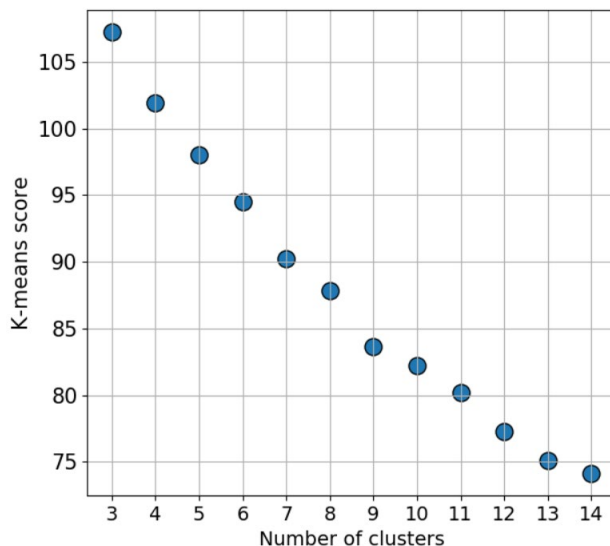
Рис. 2. Графики зависимости значений метрик от числа кластеров
