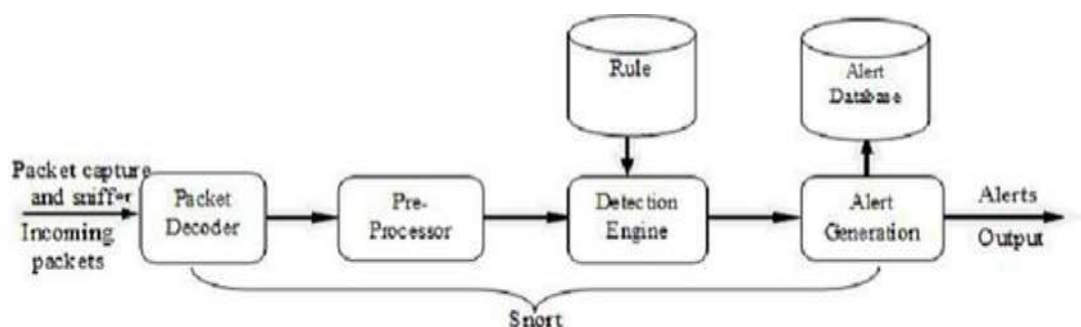
Рис. 1. Архитектура системы Snort IDS
