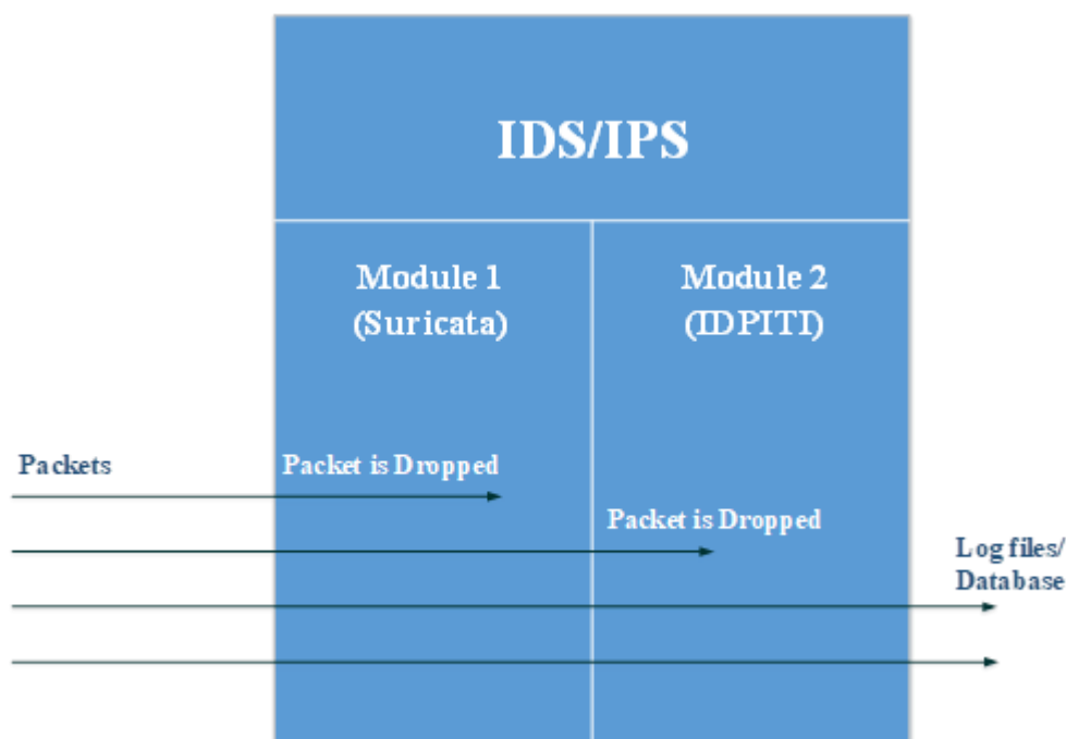
Рис. 4. Предлагаемая модель системы IDS / IPS
