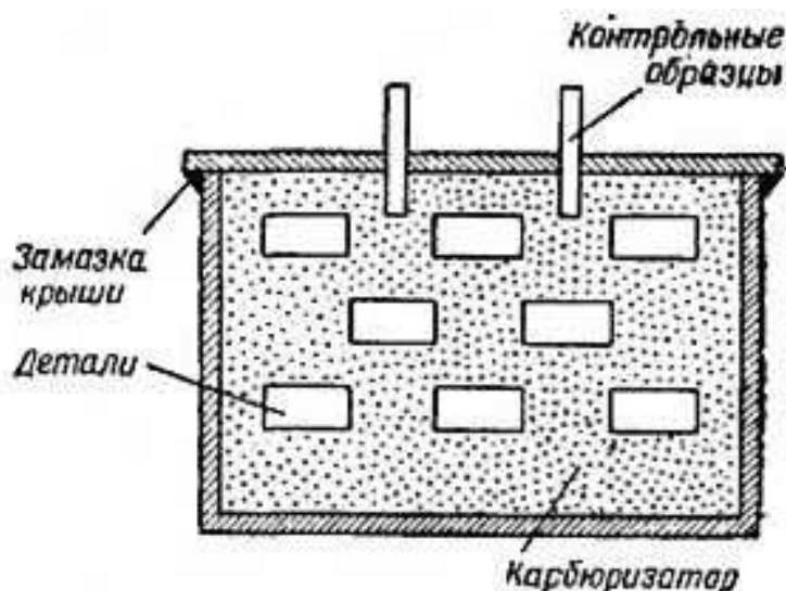
Рис. 2. Цементационный ящик с деталями
