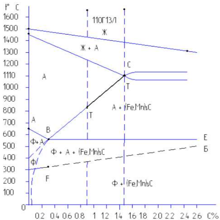
Рис. 3. Диаграмма Fe-Mn (13%)-C
