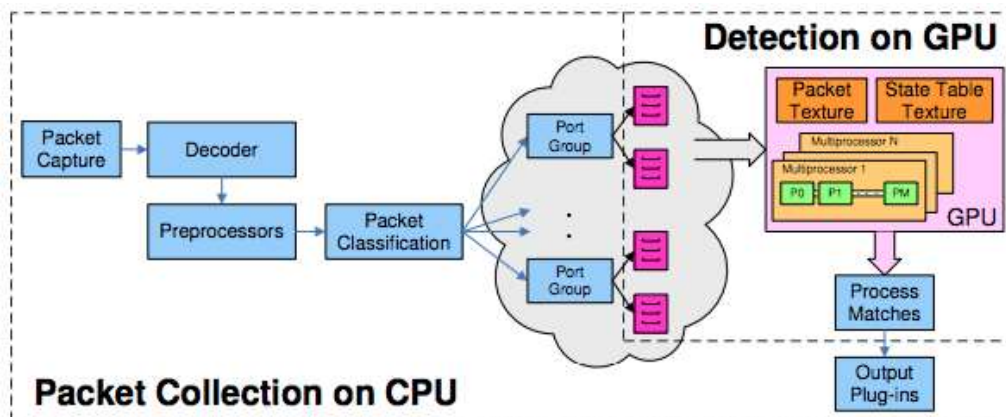
Рис. 6. Архитектура Snort
