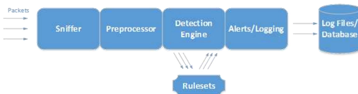
Рис. 2. Архитектура Suricata
