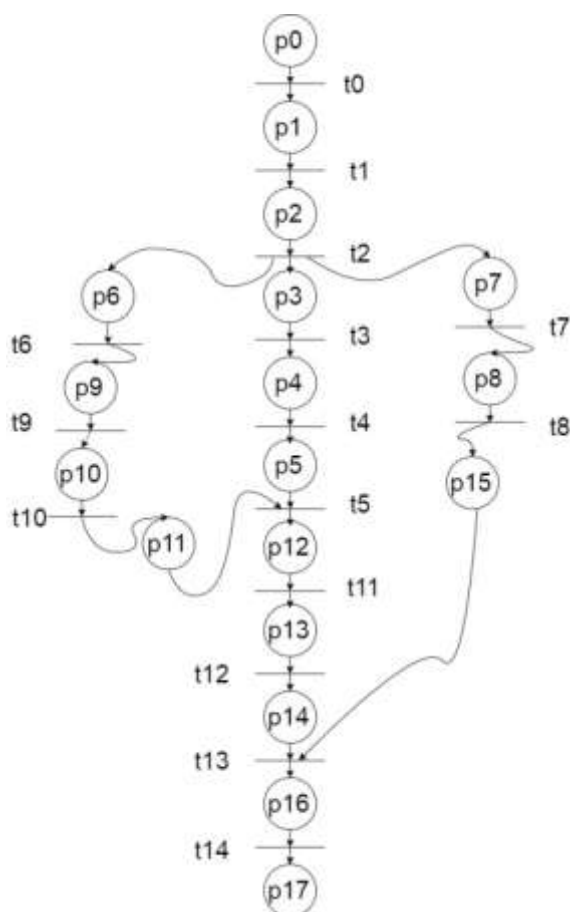
Рис. 2. Динамическая сетевая модель планирования
