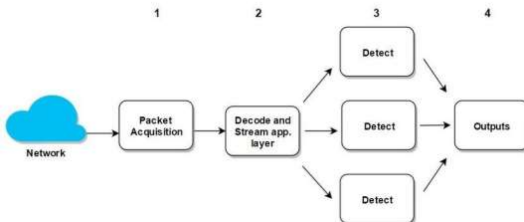
Рис. 3. Многопоточная операционная архитектура Suricata
