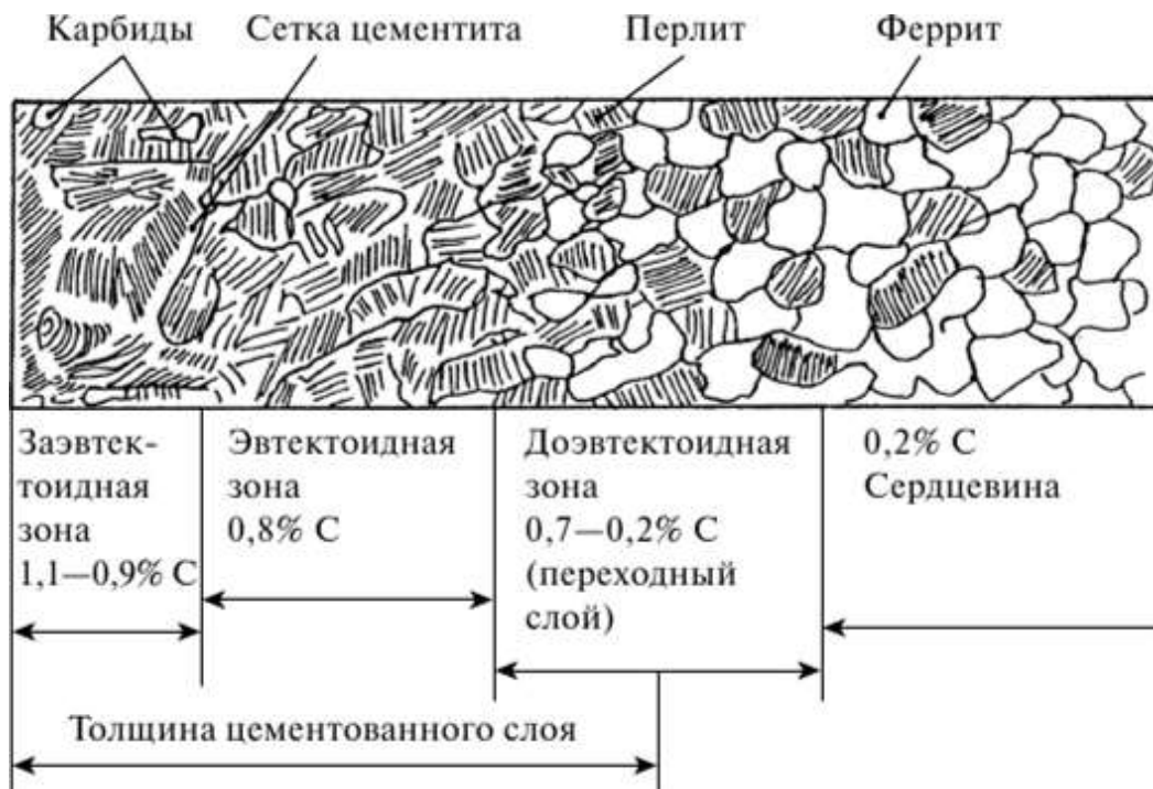
Рис. 1. Структура цементированной стали
