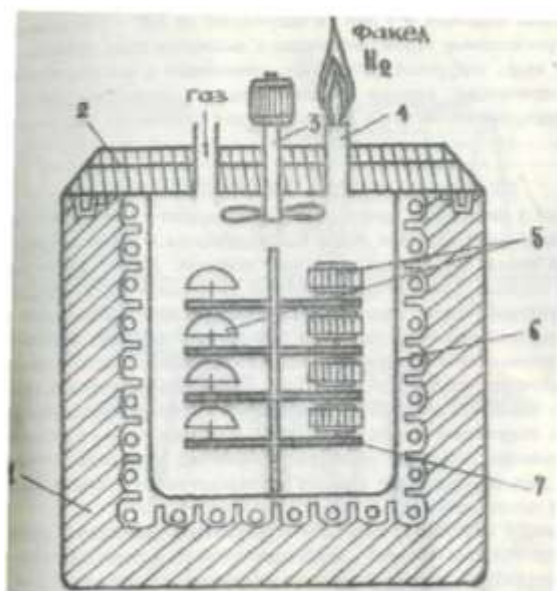
Рис. 4. Схема процесса газовой цементации
