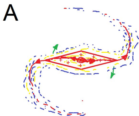
Рис. 4. А - Схема движения вещества. Б - NGC 1300 (ESO 547-31, MCG -3-9-18, UGCA 66, IRAS03174-1935, PGC 12412) – спиральная галактика с перемычкой, находится на расстоянии около 60 миллионов световых лет в созвездии Эридан
