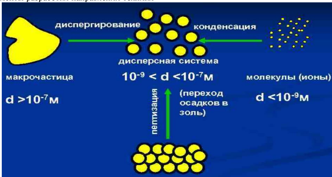
Рис. 2. Схема получения дисперсных систем [3]
