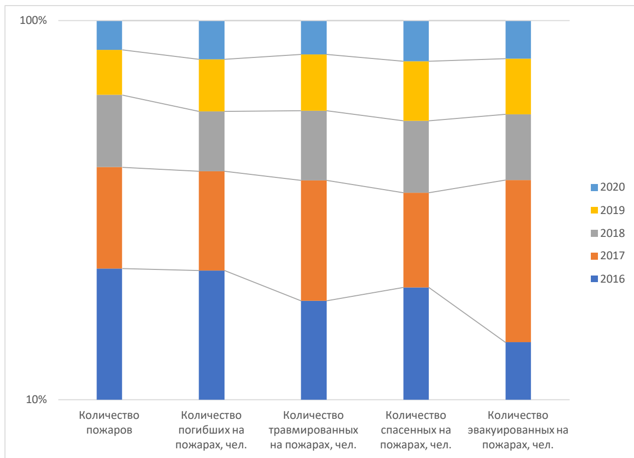
Рис. 2. Статистика количества и последствий пожаров на территории Московской области
