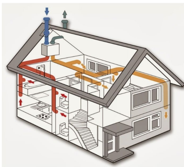
Рис. 1. Система естественной вытяжки
