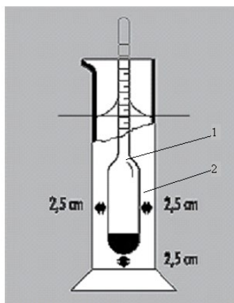
Рис. 1. Установка для определения плотности растворителя (слева - фотография, справа - схематический чертеж):
