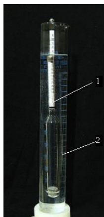
Рис. 1. Установка для определения плотности растворителя (слева - фотография, справа - схематический чертеж):
