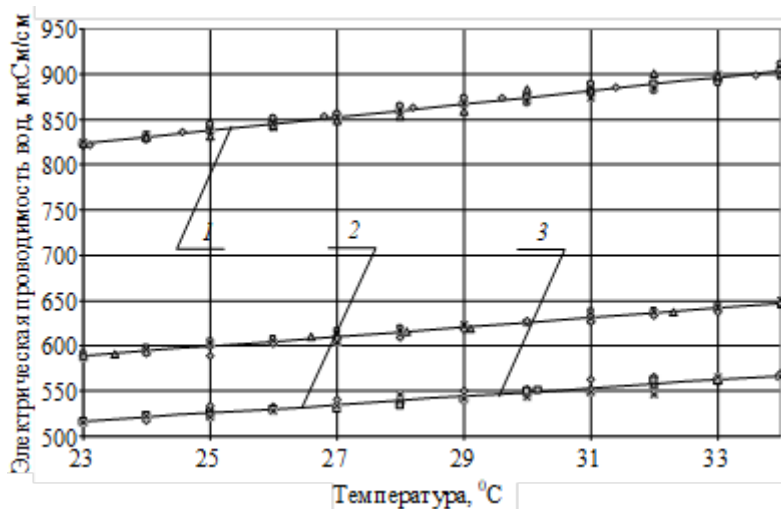
Рис. 5. Электрическая проводимость вод различной кластерной структуры при различных температурах при введении нанометалла Cu: 1 – артезианская вода; 2 – артезианская вода, пропущенная через УСВР; 3 – таялая артезианская вода
