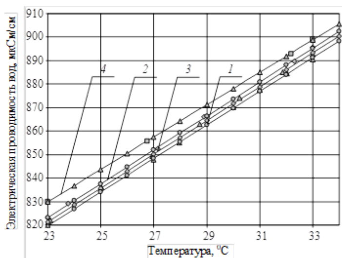
Рис. 6. Электрическая проводимость артезианской воды при введении наноструктурированных металлов при различных температурах: 1 – артезианская вода; 2 – артезианская вода с нано-Fe; 3 – артезианская вода с нано-Cu; 4 – артезианская вода с нано-Ni
