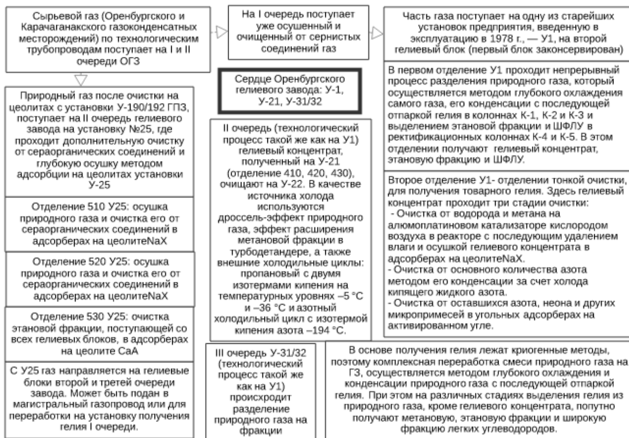
Рис. 4. Краткая схема технологии производства на ОГЗ
