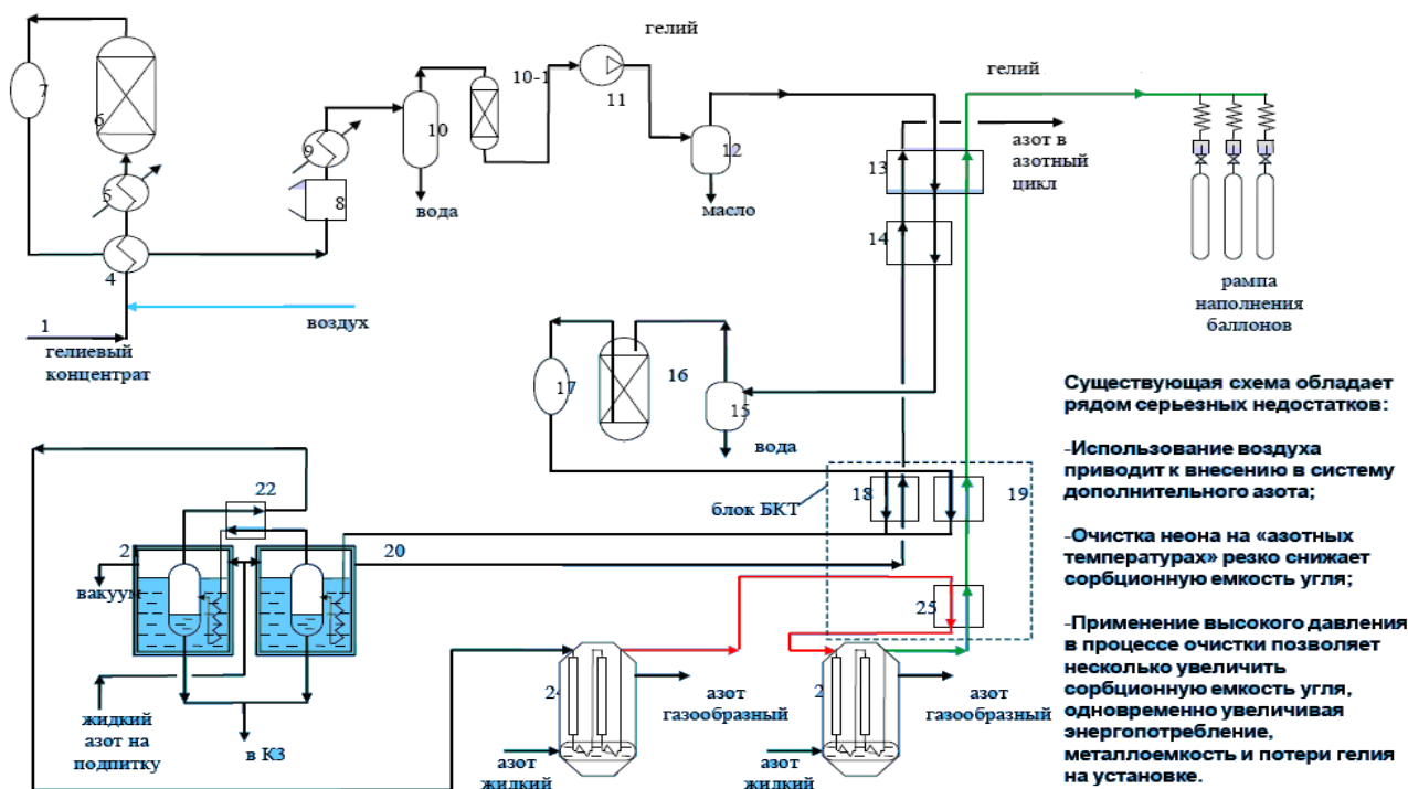
Рис. 5. Существующая схема тонкой очистки гелиевого концентрата на ОГЗ
