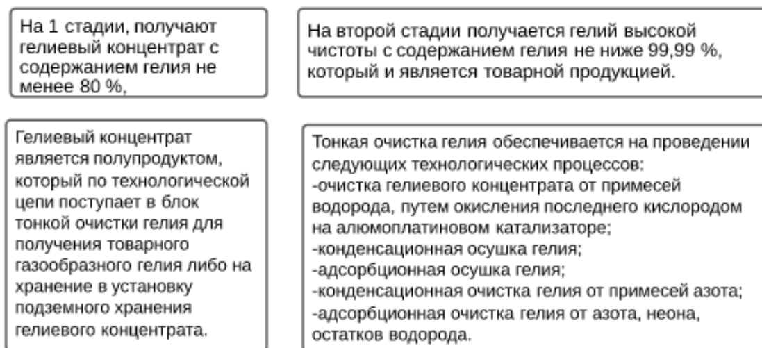
Рис. 3. Стадии производства газообразного гелия
