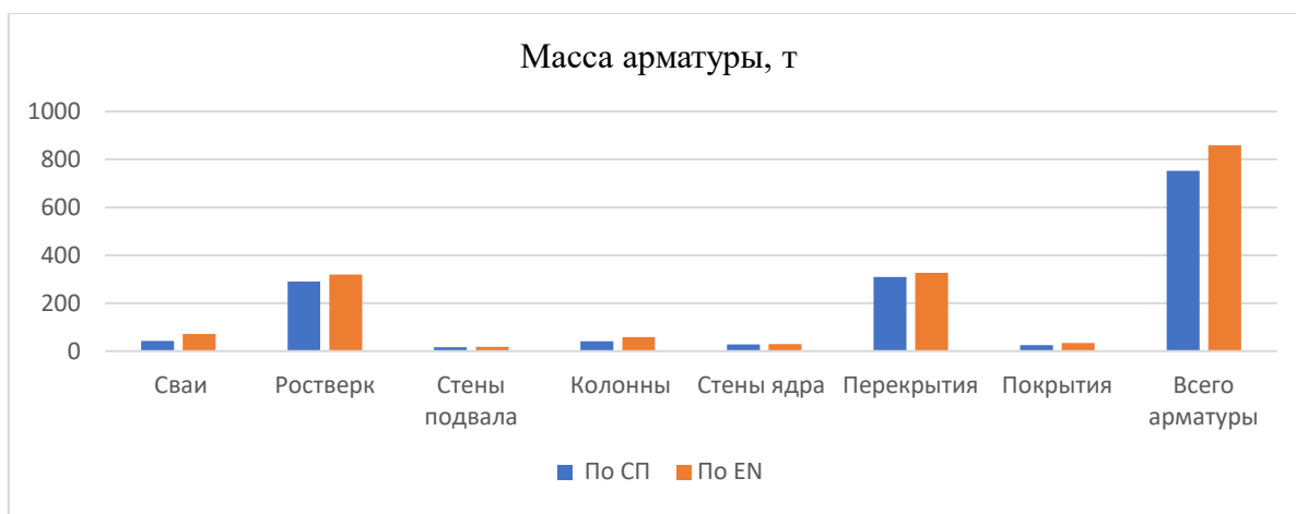
Рис. 2. Сравнения расхода арматуры по массе на железобетонный каркас
