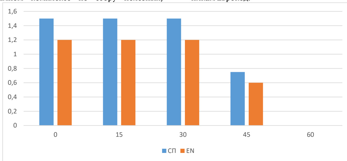
Рис. 1. Сравнение снеговой нагрузки на односкатное покрытие
