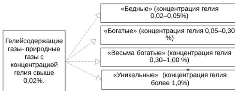
Рис. 1. Принятая в мировой практике классификация гелийсодержащих газов
