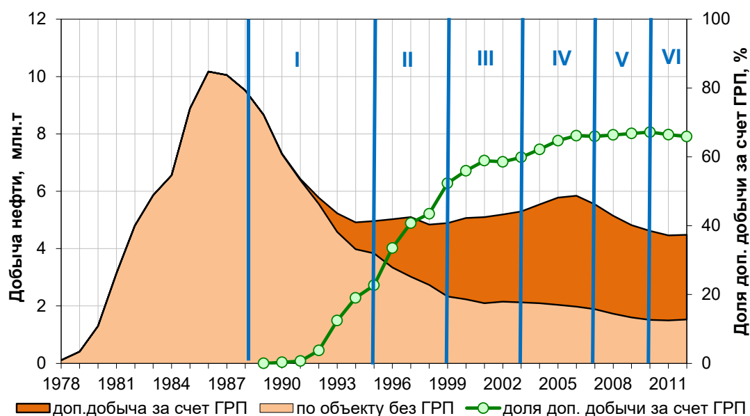
Рис. 1. Динамика изменения дополнительной добычи нефти по годам на объекте БВ8
