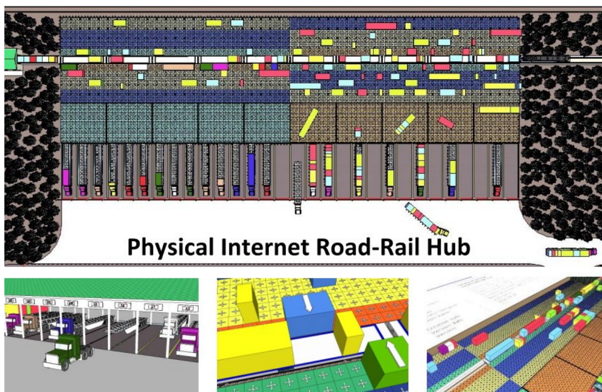
Рис. 4. Использование модульности унитарных и составных п-контейнеров для построения новых хабов «железная дорога – автомобиль» [4]
