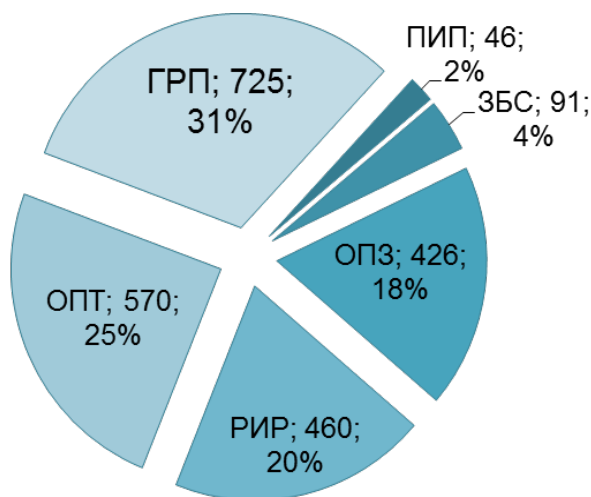
Рис. 1. Сопоставление проект/факт количества и удельной доп. добыче нефти по видам ГТМ
