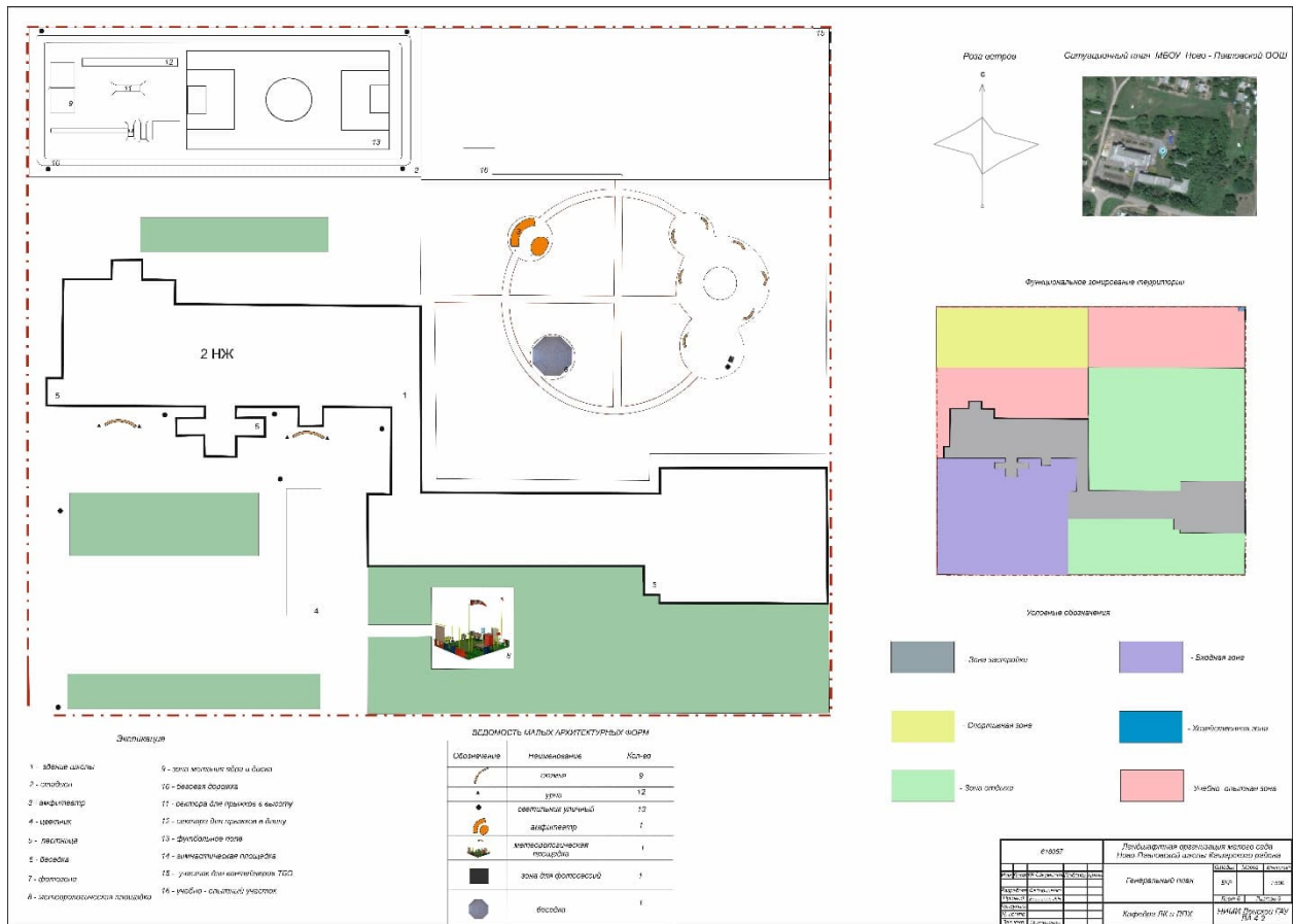
Рис. 1. Генеральный план
