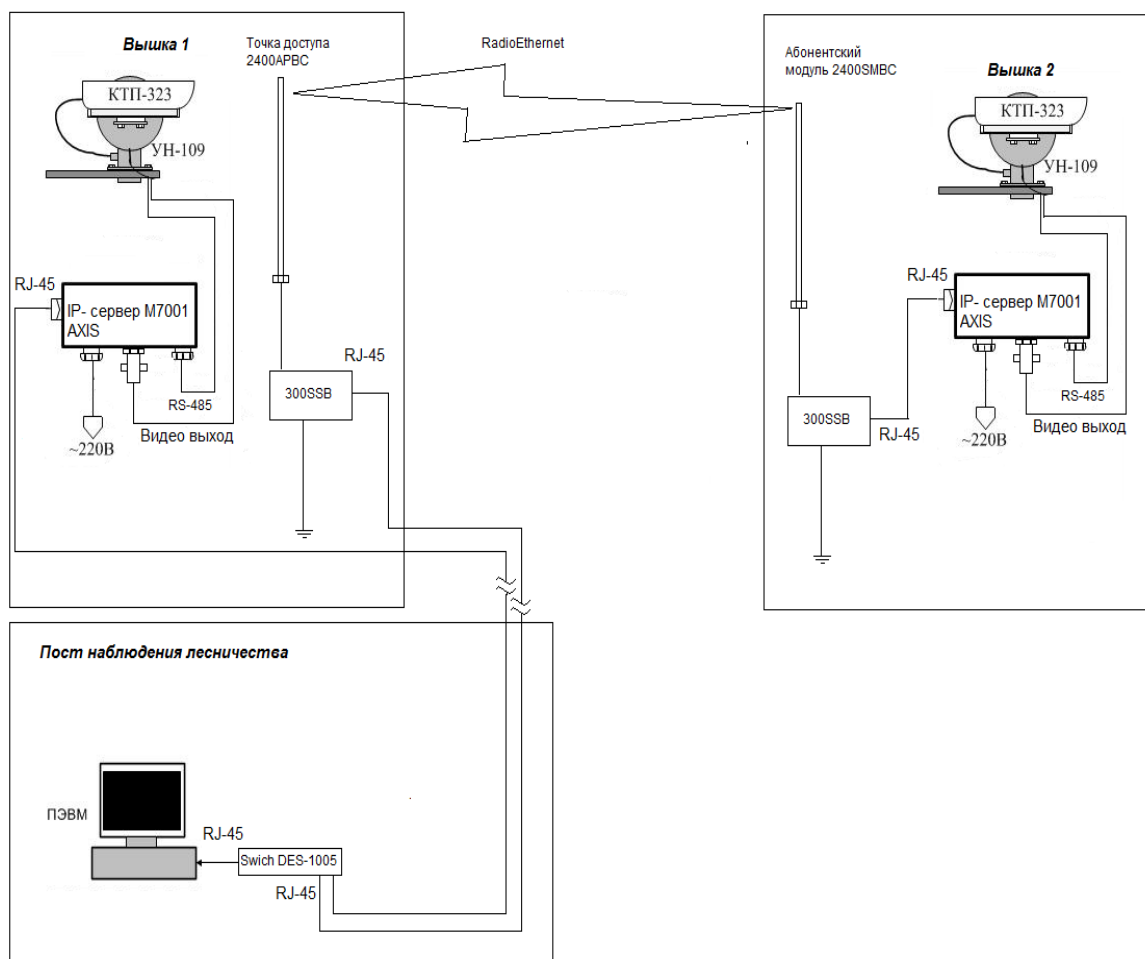
Рис. Структурная схема телевизионной системы обнаружения возгораний в лесу
