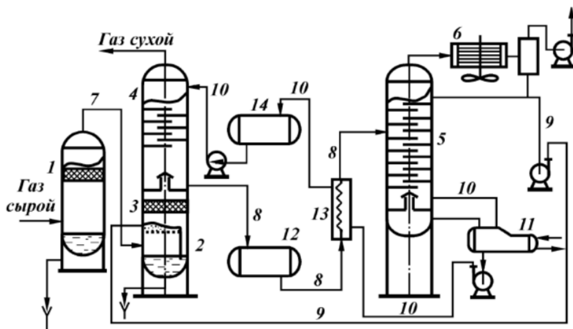
Рис. 2. Технологическая схема осушки природного газа
