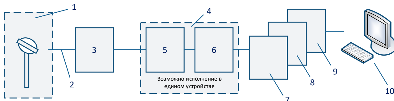
Рис. 3. Канал измерения температуры: 1 – первичный преобразователь температуры; 2 – кабельная линия связи; 3 – клеммная коробка; 4 – вторичные преобразователи; 5 – барьер искробезопасности (БИЗ); 6 – нормирующий преобразователь; 7 – плата АЦП; 8 – контроллер; 9 – сетевой интерфейс; 10 – АРМ оператора
