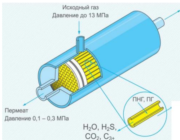
Рис. 3. Мембранные установки подготовки газа
