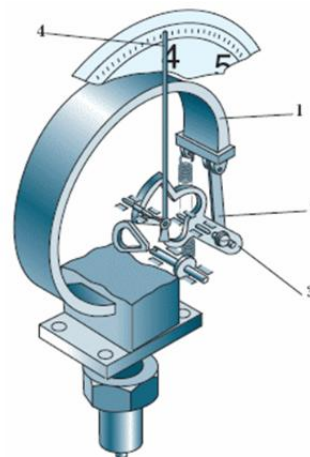
Рис. 2. Устройство пружинного манометра
