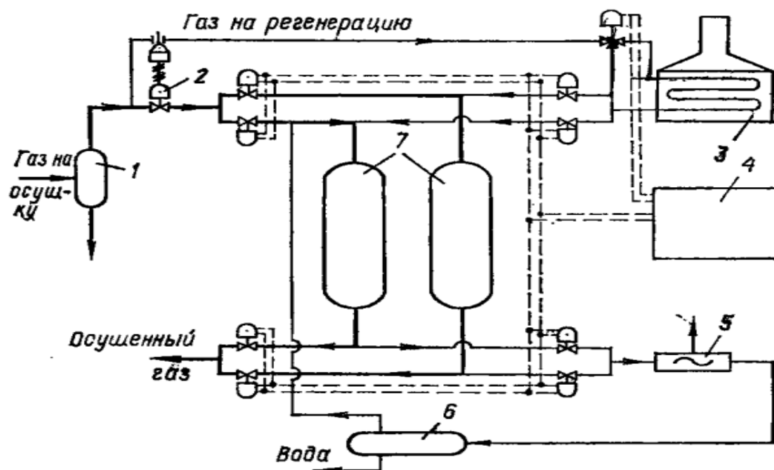
Рис. 1. Схема установки адсорбционной осушки газа
