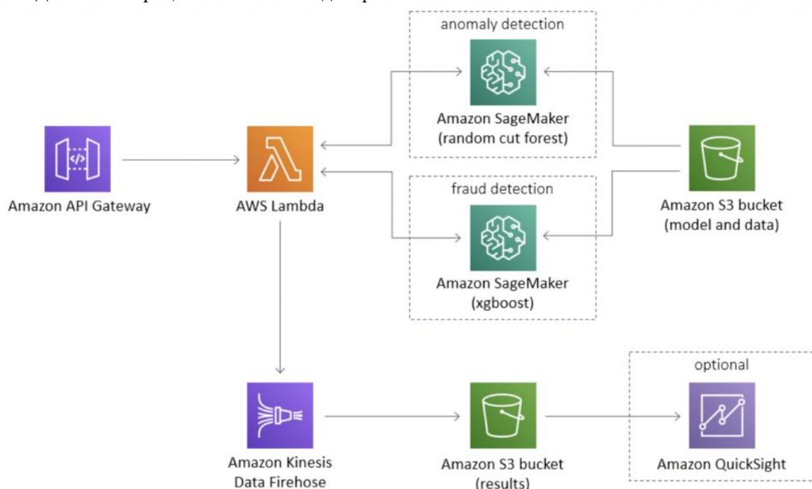
Рис. 2. Потоковая архитектура онлайн-скоринга транзакций на AWS: Kinesis → SageMaker (RCF, XGBoost) → S3/QuickSight [3]
