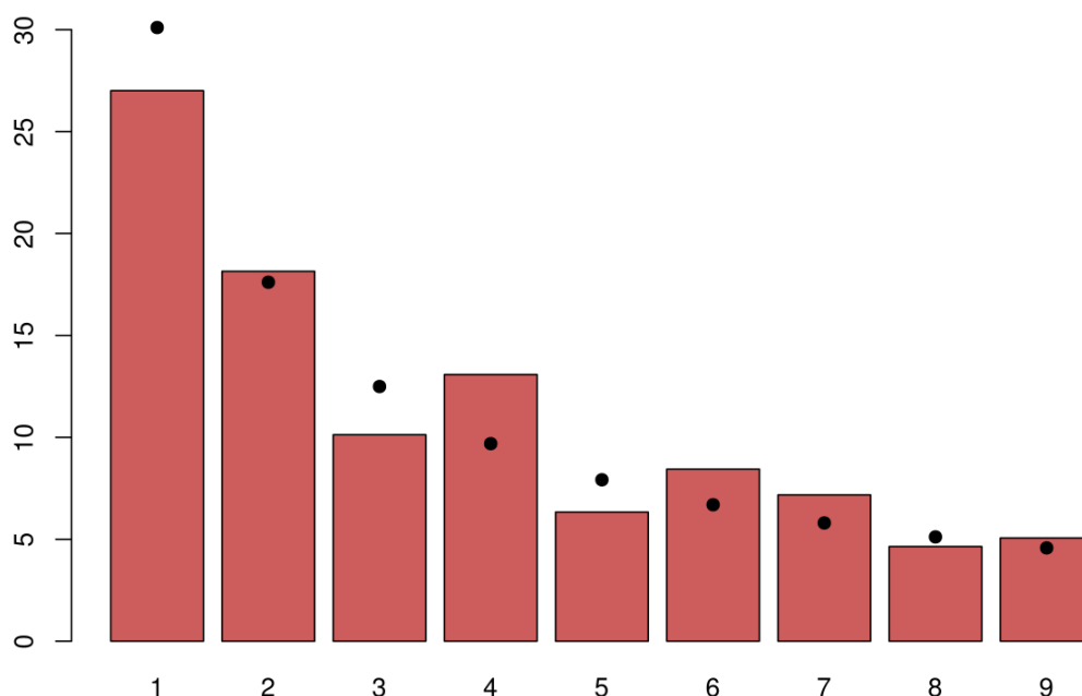
Рис. 1. Ожидаемые частоты первой цифры по закону Бенфорда (десятичная система) [4]
