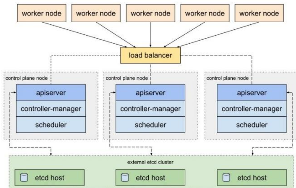
Рис. 2. Высокодоступная (НА) топология Kubernetes с внешним кластером etcd
