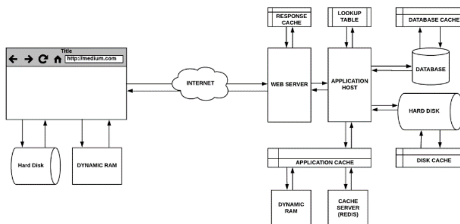
Рис. 4. Архитектура веб-приложения с многослойным кэшированием
