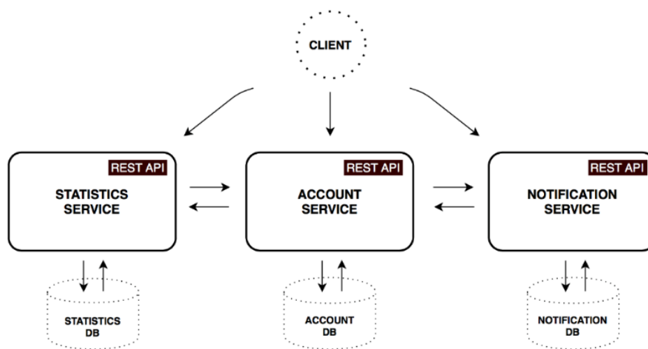
Рис. 1. Схема микросервисной архитектуры с тремя независимыми сервисами
