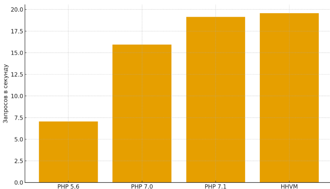
Рис. 2. Производительность Drupal 8.4.4 (запросов/с) на разных рантаймах [1]
