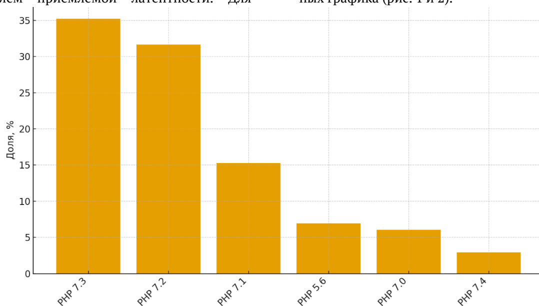
Рис. 1. Распределение версий PHP в экосистеме Packagist (Composer) [5]
