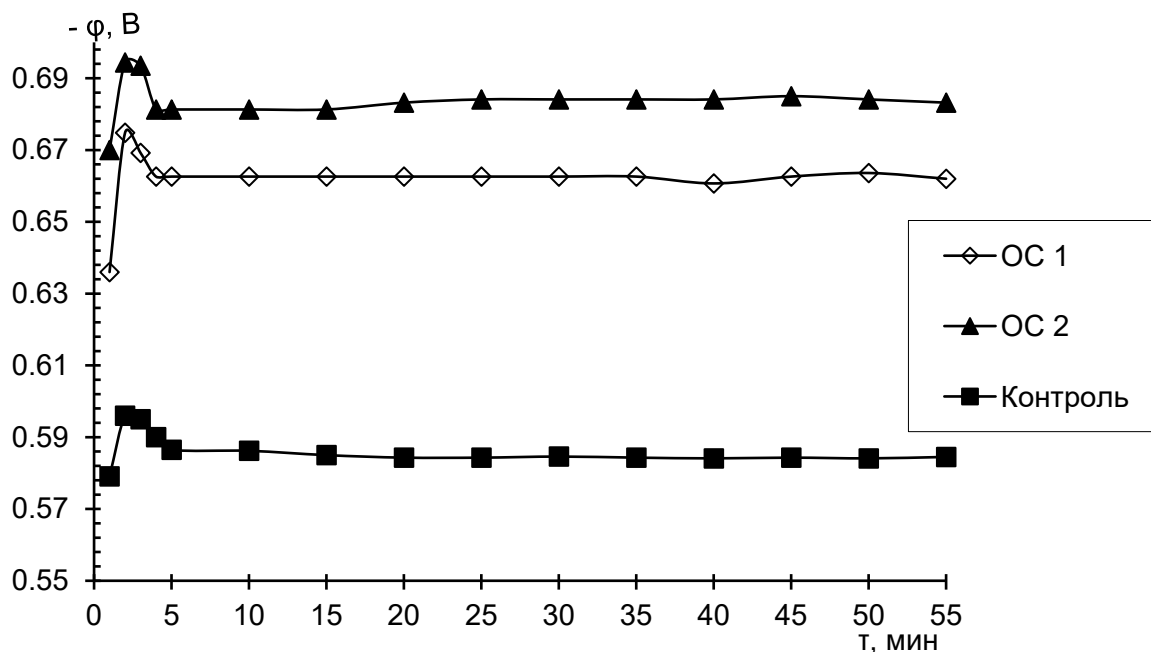
Рис. 1. Зависимость потенциала катода от времени при электроосаждении цинка D_k = 0,5 А/дм 2 в присутствии 5 ммоль/л ОС
