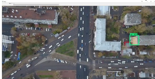
Рис. 8. Результат работы нейронной сети с изображением с не подобранным масштабом
