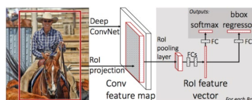
Рис. 4. Схема сети Fast R-CNN
