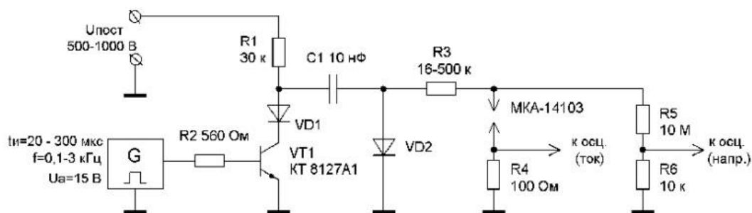
Рис. 1. Электрическая принципиальная схема генератора импульсного напряжения
