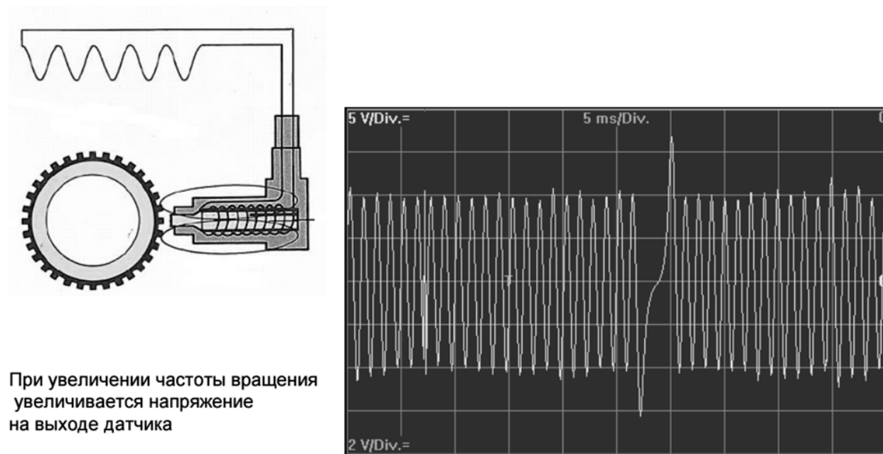
Рис. 1. Работа датчика скорости колес автомобиля
