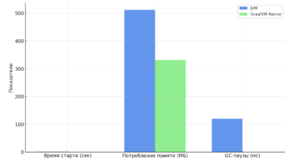
Рис. 3. Сравнение производительности JVM и GraalVM Native
