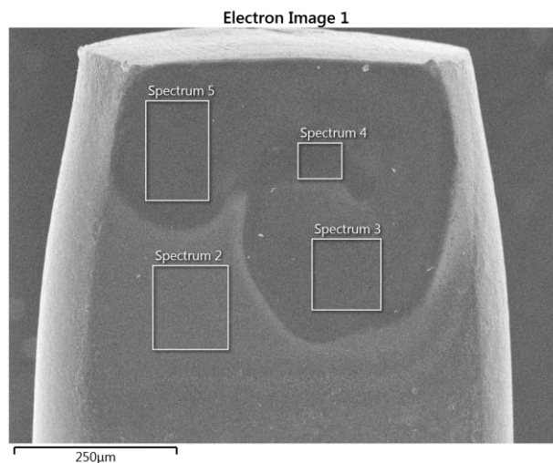
Рис. 6. Электронное изображение контакта геркона
