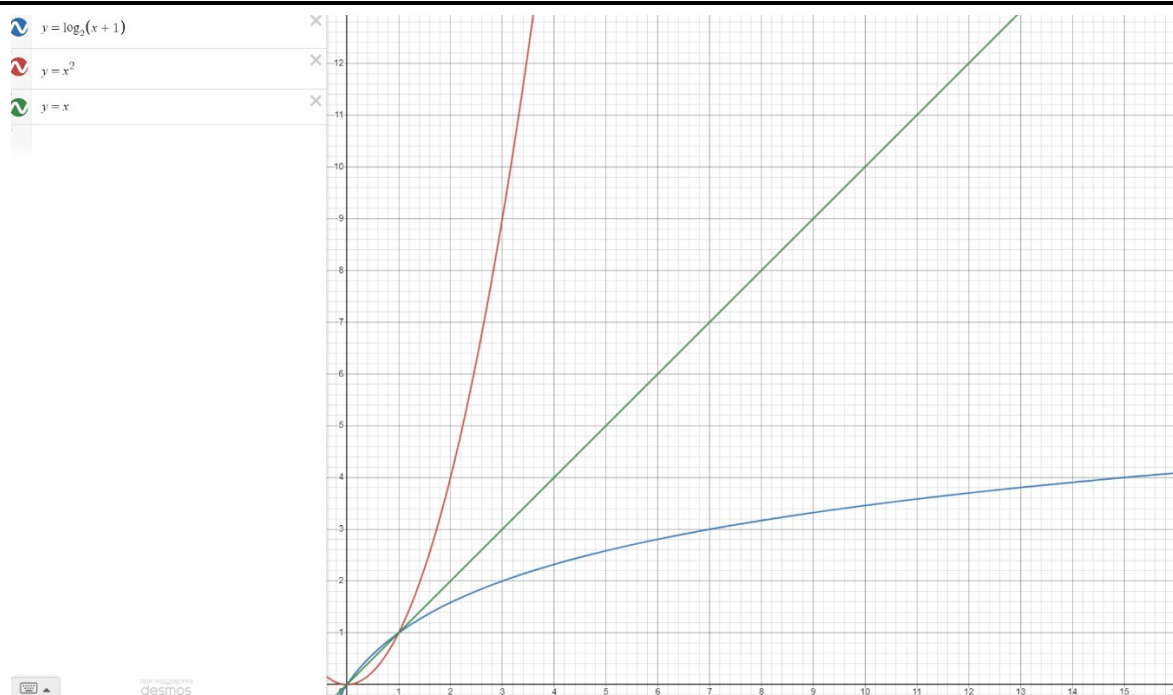
Рис. 3. График затрат времени( y ) при количестве элементов поиска ( x ) у алгоритмов с логарифмической сложностью (синяя линия), линейной сложностью (зеленая линия), квадратичной сложностью (красная линия)
