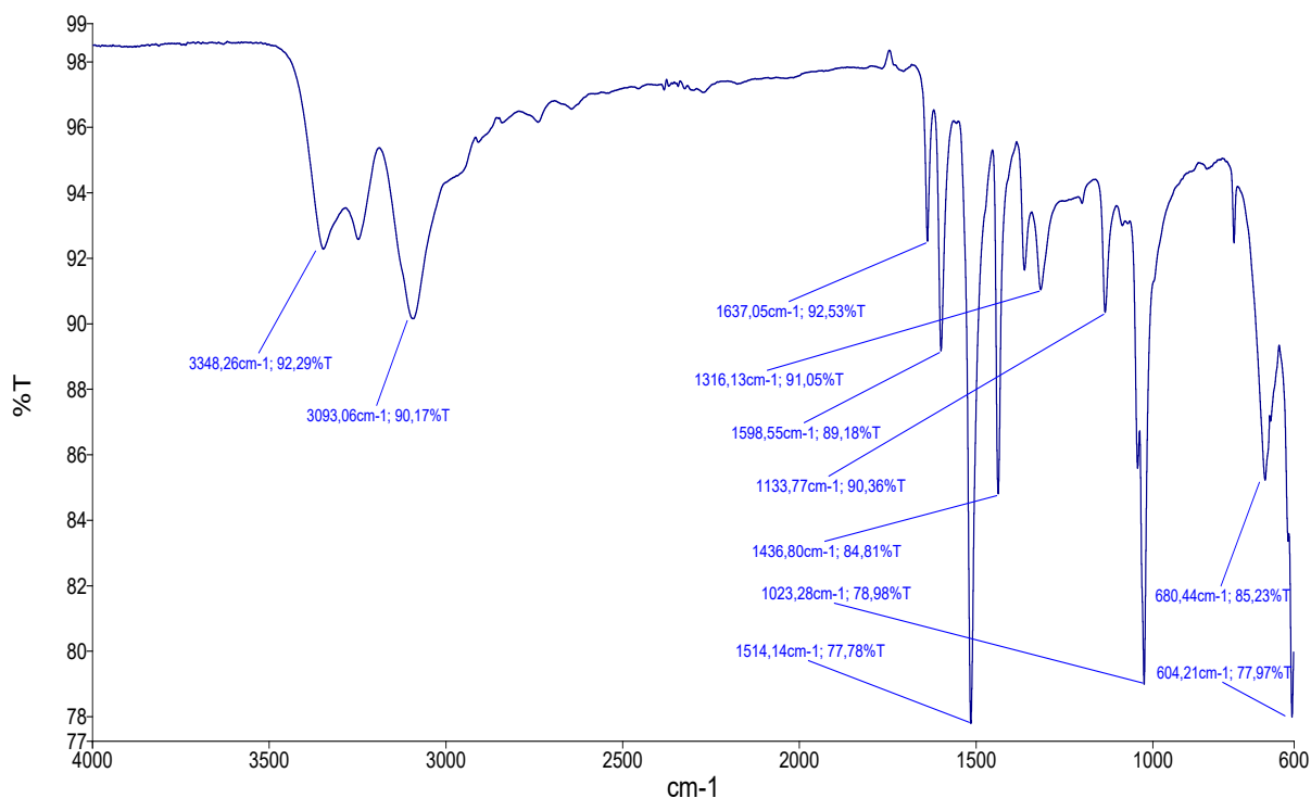
Рис. 1. ИК-спектр 2-бром-6-винилимидазо[2,1- b ][1,3,4]тиadiaзола ( 2 )
