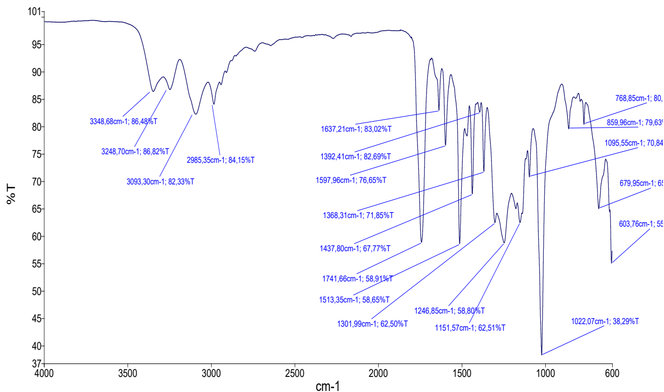
Рис. 2. ИК-спектр этил 2-бromo-6-гидроксиимидазо-[2,1-b][1,3,4]-тиадiazол карбоксилата (3)
