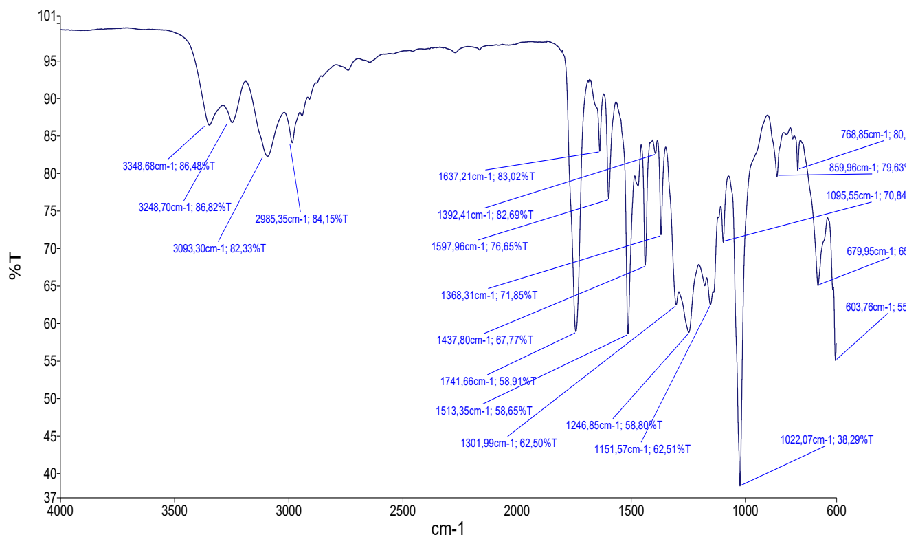
Рис. 2. ИК-спектр этил 2-бromo-6-гидроксиимидазо-[2,1-b][1,3,4]-тиадиазол карбоксилата (3)
