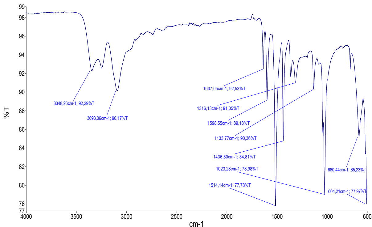
Рис. 1. ИК-спектр 2-бром-6-винилимидазо[2,1- b ][1,3,4]тиадиазола (2)
