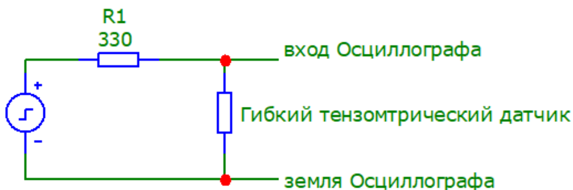
Рис. 3. Принципиальная схема цепи для проверки теории
