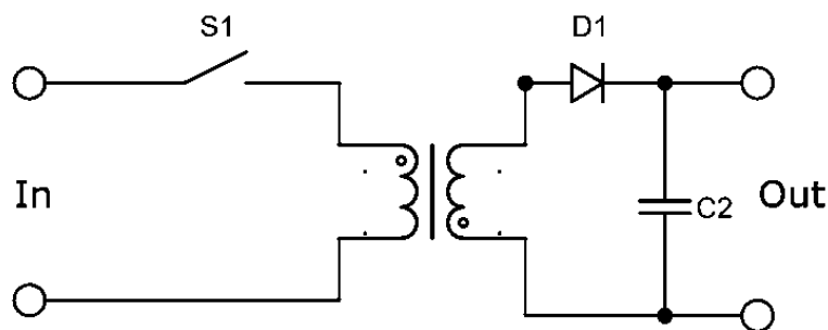
Рис. 6. Топология Flyback
