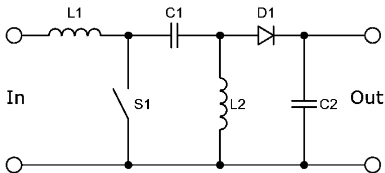
Рис. 4. Топология SEPIC
