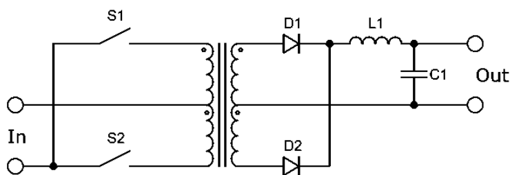
Рис. 9. Топология Push-Pull
