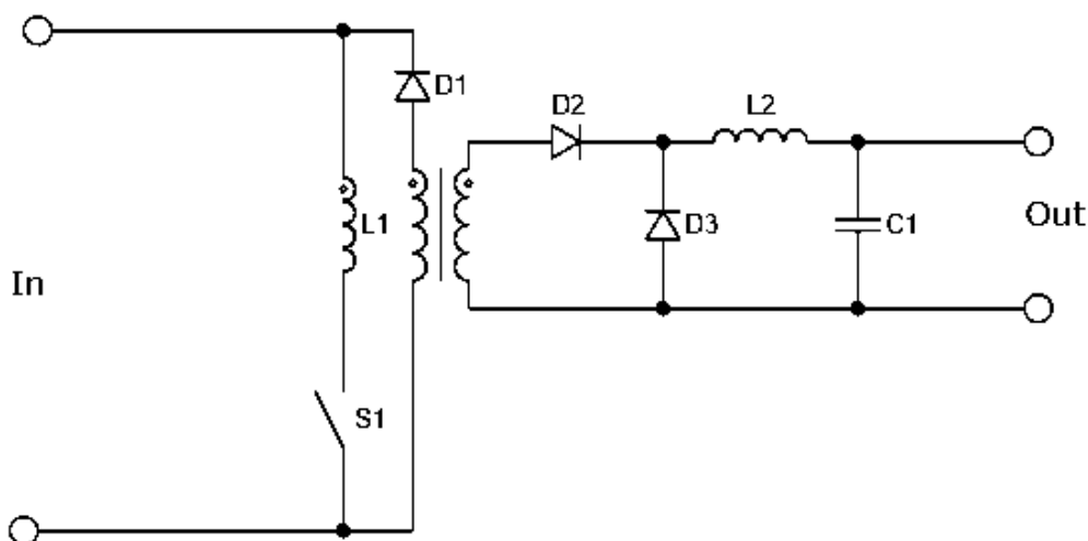
Рис. 7. Топология Forward
