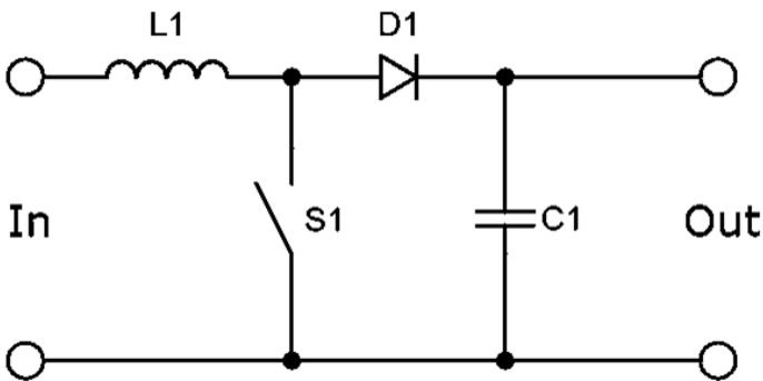
Рис. 2. Топология Boost
