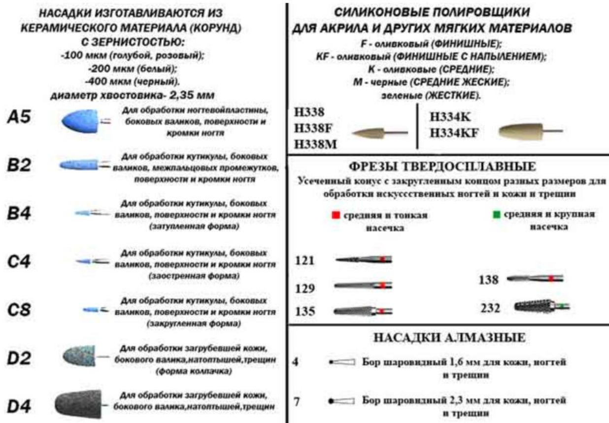
Рис. Основные типы фрез
