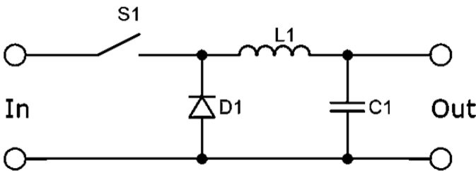
Рис. 1. Топология Buck
