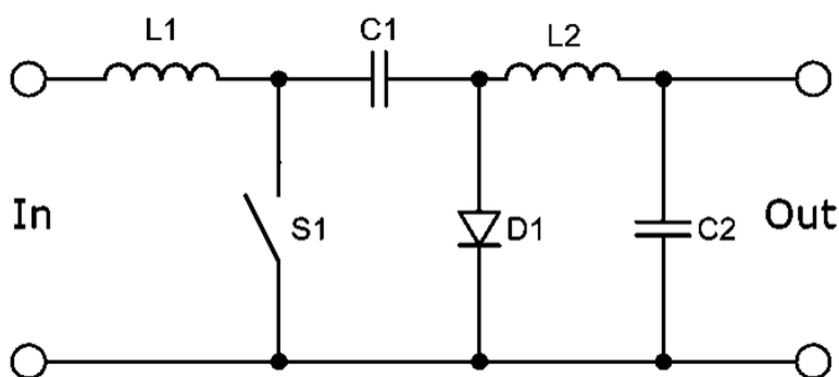
Рис. 5. Топология Cuk
