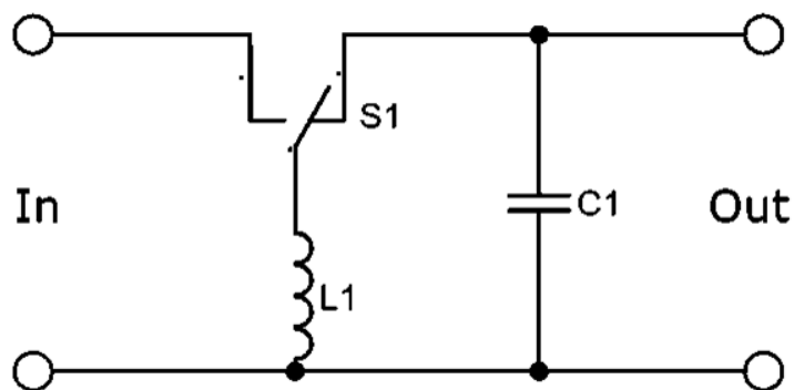
Рис. 3. Топология Buck-Boost
