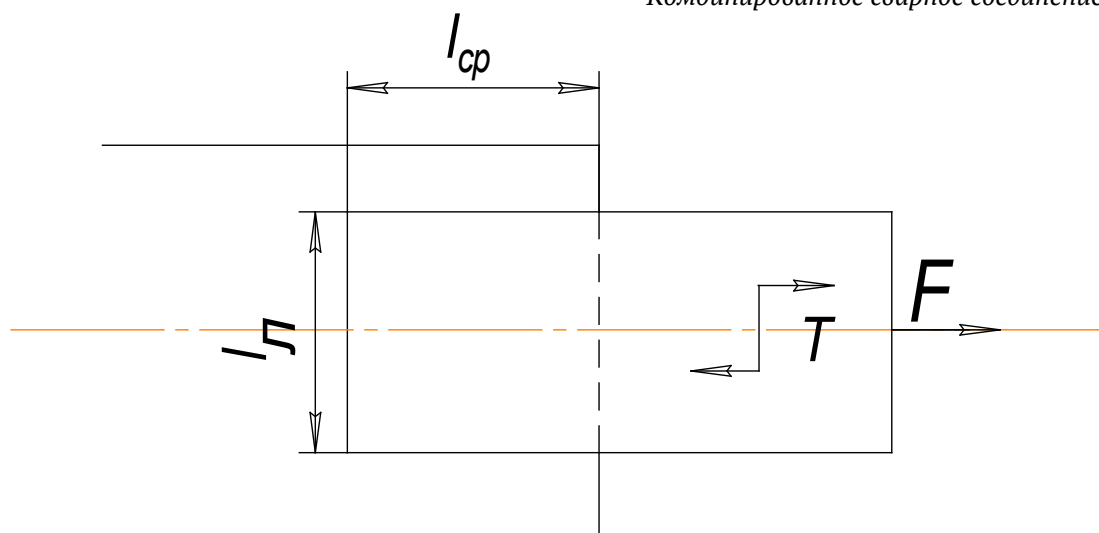
Рис. 4. Комбинированное сварное соединение
