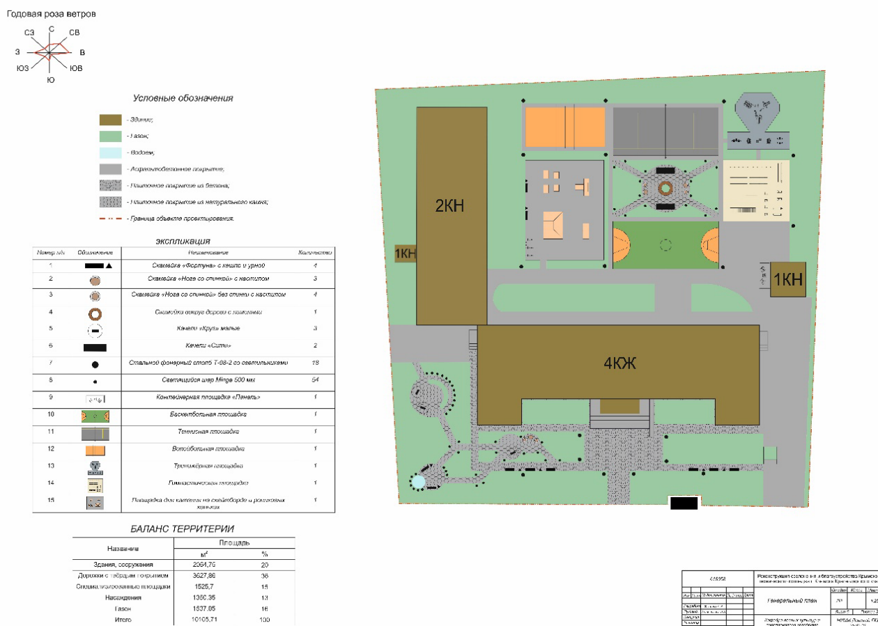
Рис. 1. Генеральный план
