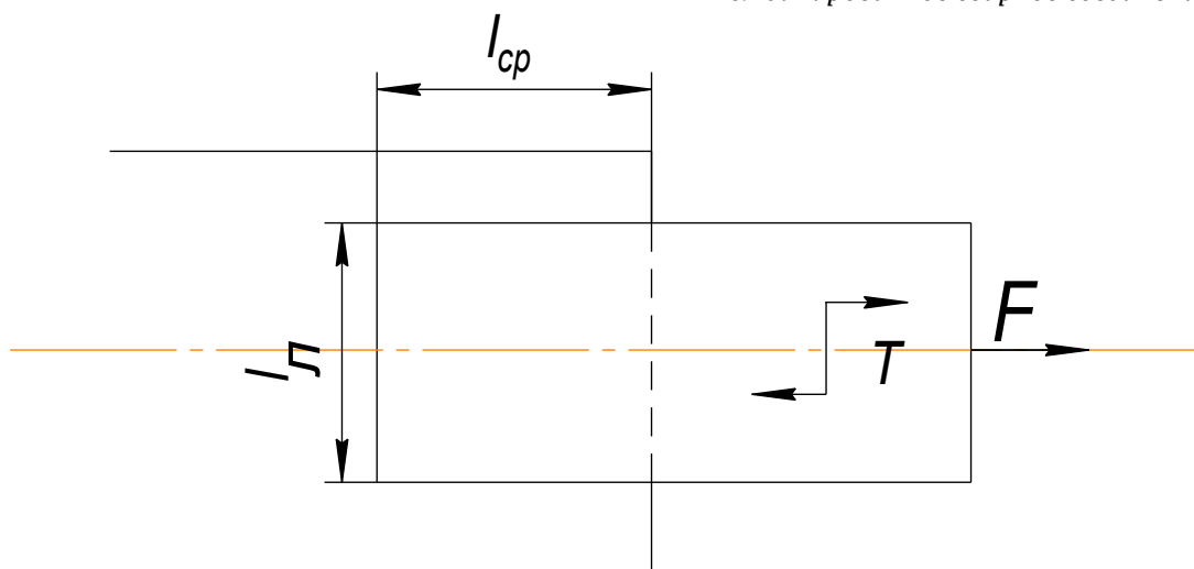
Рис. 4. Комбинированное сварное соединение
