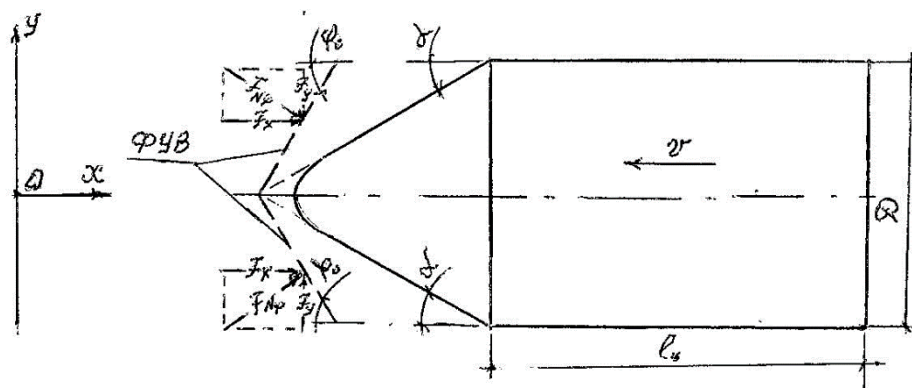
Рис. 7. Схема сил лобового сопротивления
