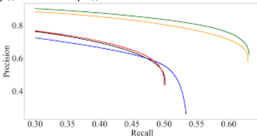
Рис. 8. Кривая P-R
