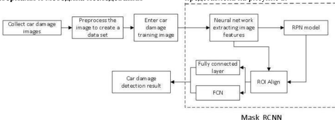
Рис. 1. Фреймворк системы обнаружения повреждений автомобилей
