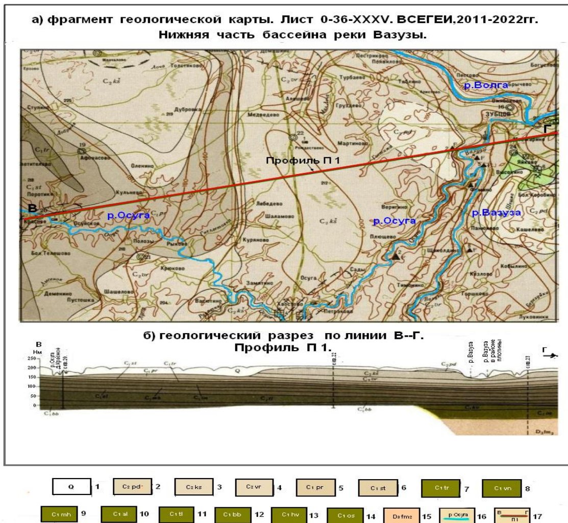
Рис. 5. Фрагмент геологической карты, охватывающий нижнюю часть бассейна реки Вазузы (а), лист 0-36-XXXV, ВСЕГЕИ, 2011-2022 гг. [2], и геологический разрез к этой карте по линии В-Г, профиль П1 (б). Условные обозначения: 1 – четвертичные отложения; 2 – подольский горизонт, известняки; 3 – каширский горизонт, известняки; 3 – верейский горизонт, глины; 5 – протвинский горизонт, известняки; 6 – стешевский горизонт, глины, мергели; 7 – тарусский горизонт, известняки; 8 – веневский горизонт, известняки; 9 – михайловский горизонт, известняки; 10 – алексинский горизонт, известняки; 11 – тульский горизонт, известняки; 12 – бобриковский горизонт, известняки; 13 – заволжский горизонт, хованский слой, доломиты, мергели, глины; 14 – заволжский горизонт, озерская толща, доломиты, мергели, глины; 15 – верхнедевонские отложения, верхнефаменский ярус, доломиты, с прослоями глин и мергелей; 16 – речная сеть до образования Вазузского водохранилища; 17 – геологический разрез по линии В-Г, профиль П1
