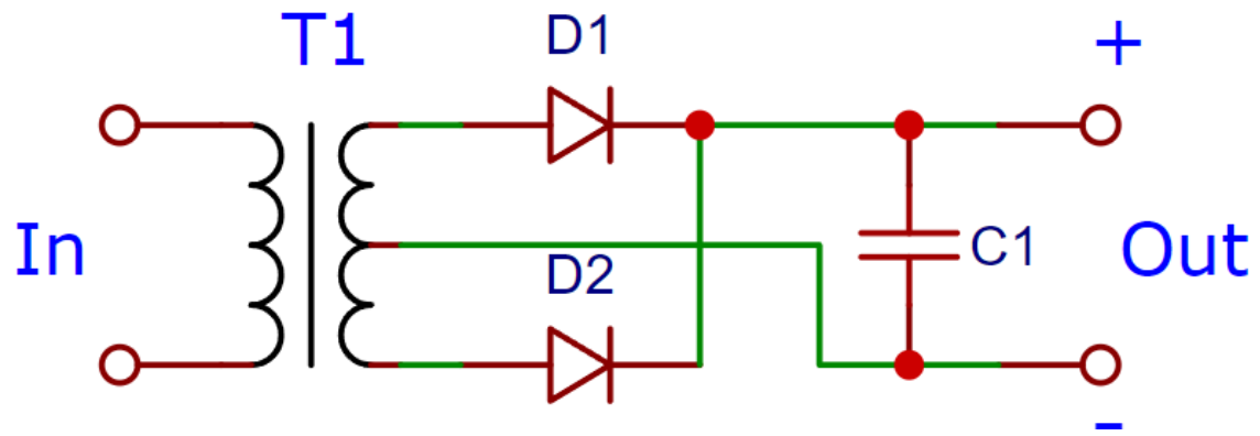
Рис. 4. Двухполупериодная схема выпрямителя
