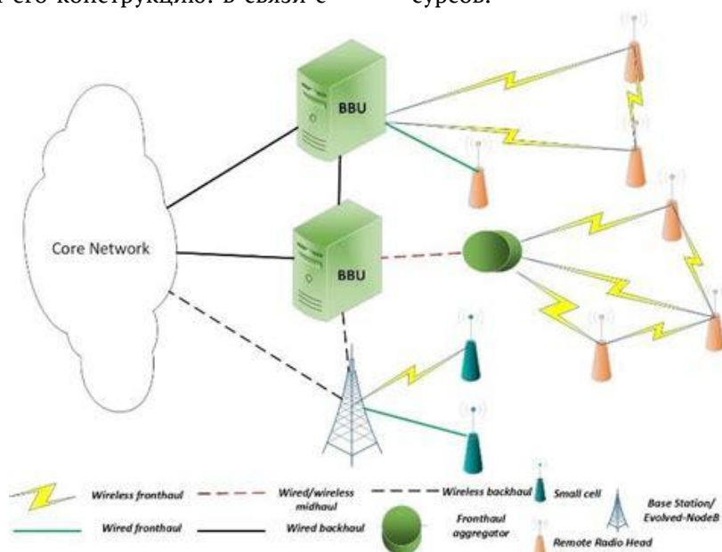
Рис. 2. Архитектура сотовой сети с разделением на фронтхол, мидхол и бэкхол сегменты
