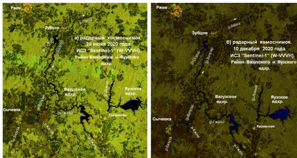
Рис. 13. Радарные космические снимки района Вазузского и Яузского водохранилищ за летний (а) и зимний (б) периоды. ИСЗ «Sentinel-1, W-VVVH [7]. Дата съемки: а) 20 июня 2020 года; б) 10 декабря 2020 года
