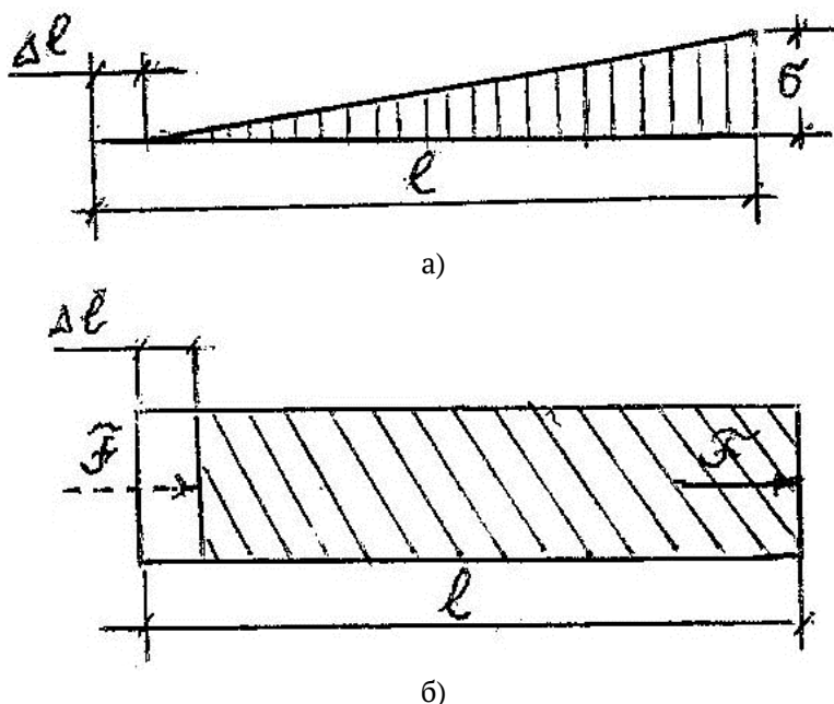
Рис. 4. Эпюры ударных напряжений
