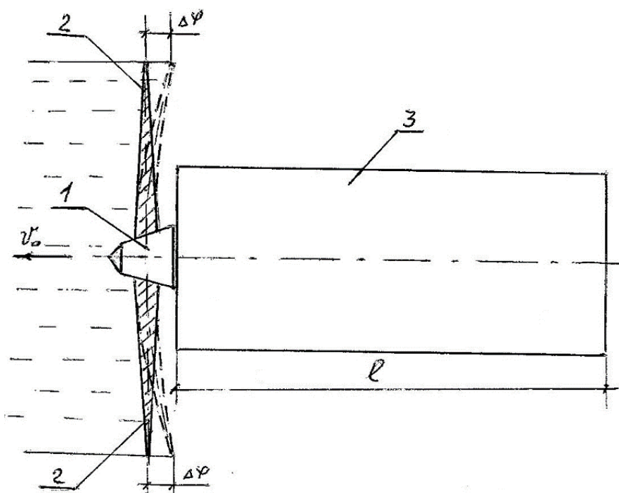
Рис. 3. Деформация прогиба лопастей гребного винта
