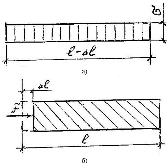
Рис. 2. Эпюра напряжений \sigma статического сжатия
