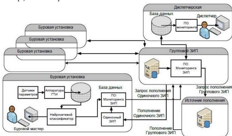
Рис. Структура системы мониторинга состояния буровых и снабжения ЗИП [1, с. 121-131]
