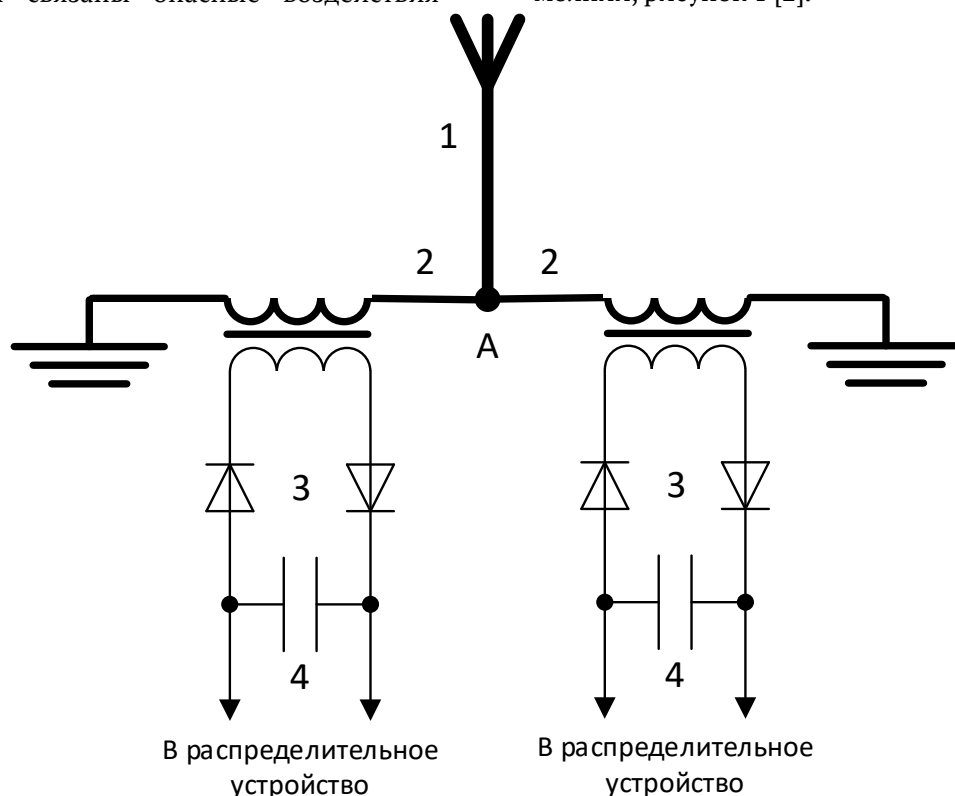
Рис. 1. Возможное устройство использования электроэнергии молнии
