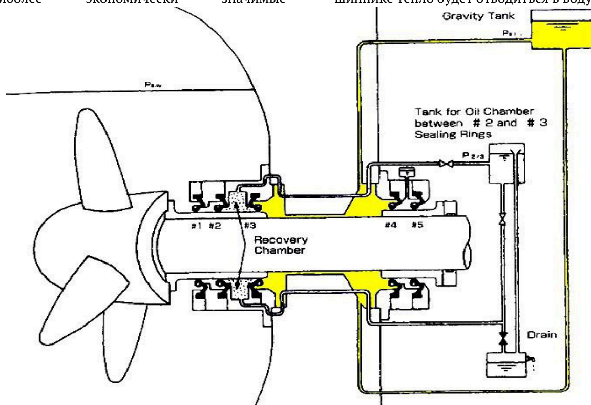
Рис. 2. Упрощённая схема дейдвудного устройства
