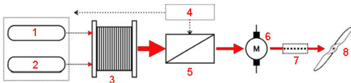
Рис. 1. Структурная схема установки: 1 – водород; 2 – кислород; 3 – топливная ячейка (РЕМ); 4 – контроллер; 5 – преобразующая электроника; 6 – мотор постоянного тока; 7 – вал мотора; 8 – пропеллер
