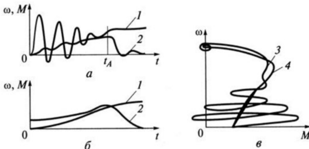
Рис. 1. Кривые переходных процессов при учете электромагнитных процессов (а), без учета электромагнитных процессов (б) и двигателя (в): 1 – графики скорости; 2 – графики момента; 3 – динамические характеристики при учете электромагнитных процессов; 4 – динамические характеристики без учета электромагнитных процессов
