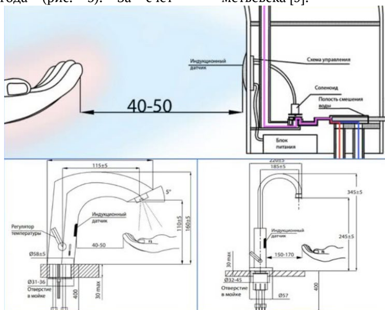
Рис. 3. Принцип работы и установка бесконтактного смесителя
