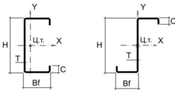
Рис. 1. Параметры С- и Z- образных профилей
