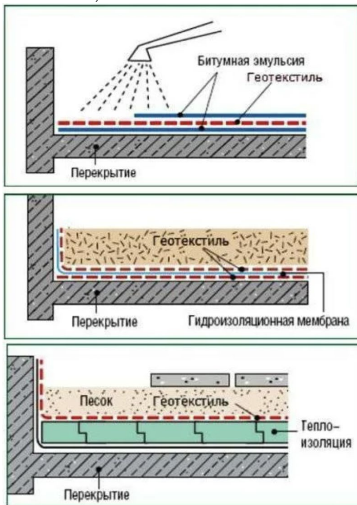
Рис. 1. Пример применения геотекстиля
