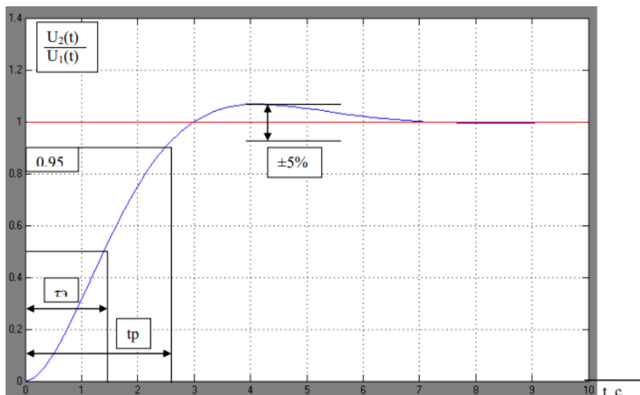
Рис. 2. Изображение переходного процесса в системе управления ракетой
