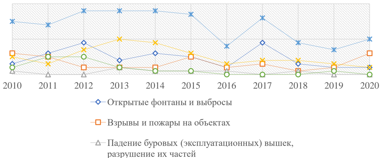
Рис. 1. Статистический анализ аварий в газодобыче и смежной отрасли (нефтедобыче) по частоте возникновения в динамике в динамике последнего десятилетия [2010/2020] (по данным Ростехнадзора)
