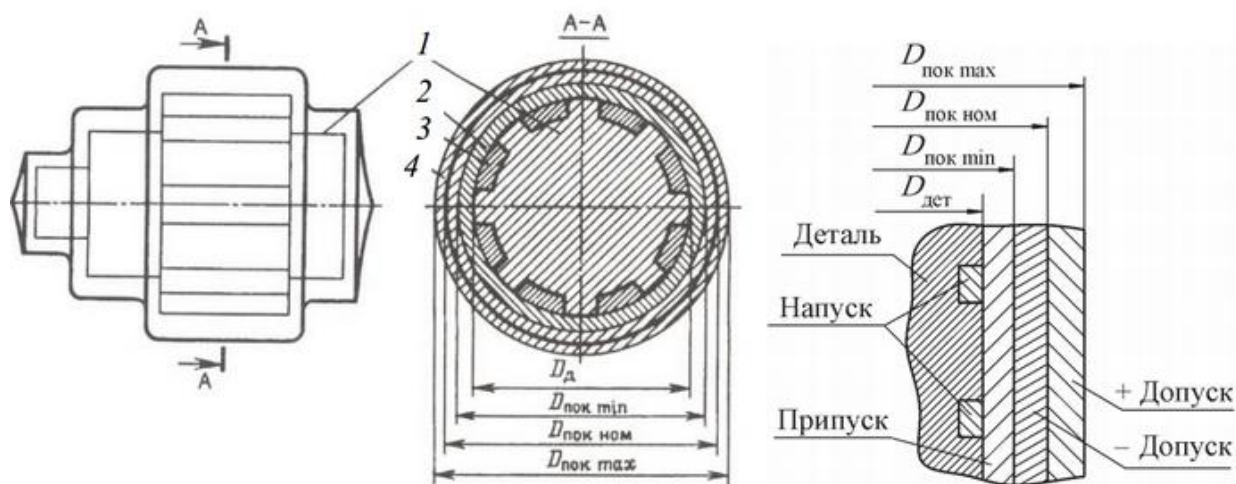
Рис. 1. Схема размеров поковки: 1 – деталь; 2 – припуск; 3 – напуск; 4 – допуск
