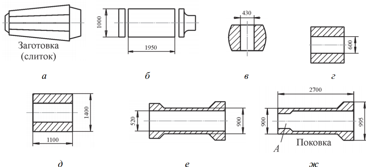
Рис. 2. Последовательность операцийковки полого цилиндра из слитка:
